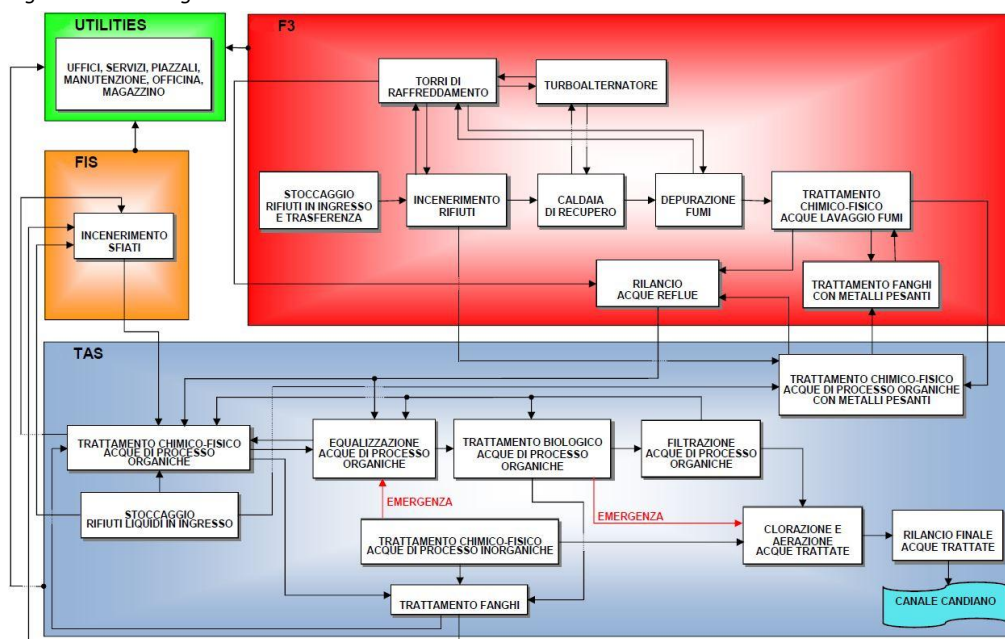
Figura 6 Schema generale del sito
