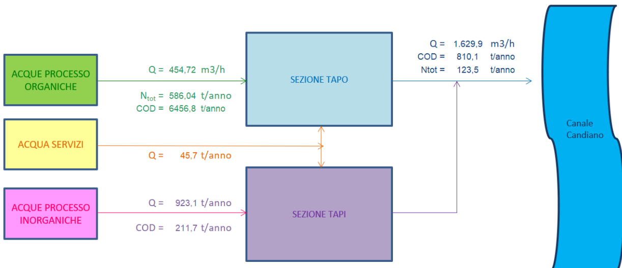
Figura 36 Bilancio impianto TAS (2025)
