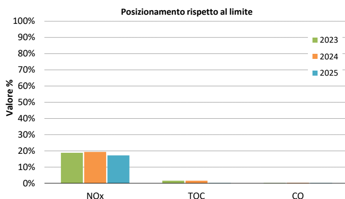
Figura 40 Andamento dell'indicatore "Posizionamento rispetto al limite" (E1)
