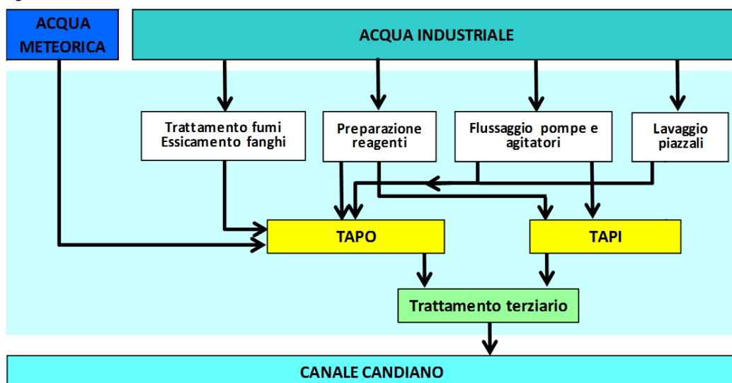
Figura 32 Ciclo idrico – TAS
