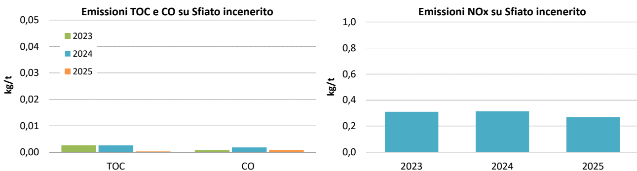
Figura 41 Andamento dell'indicatore "Fattori di emissione in atmosfera" (E1)
