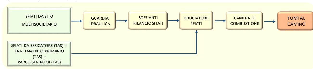
Figura 11 Ciclo produttivo (FIS)
