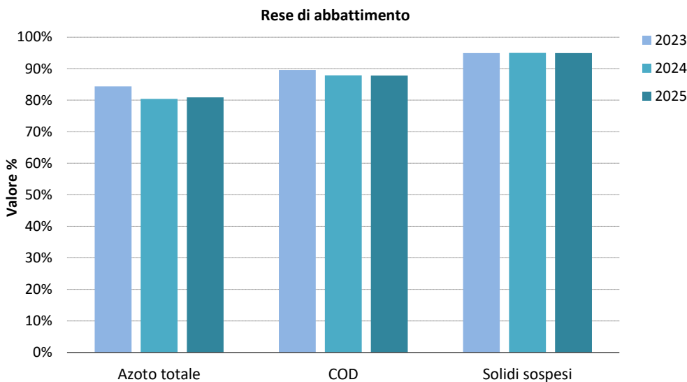
Figura 35 Andamento dell'indicatore "Efficienza di abbattimento" (TAS)
