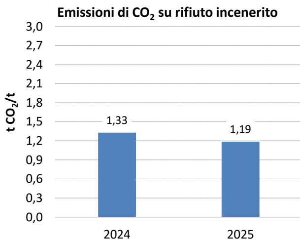
Figura 43 Andamento dell'indicatore "Fattore di emissione gas serra" (F3)
