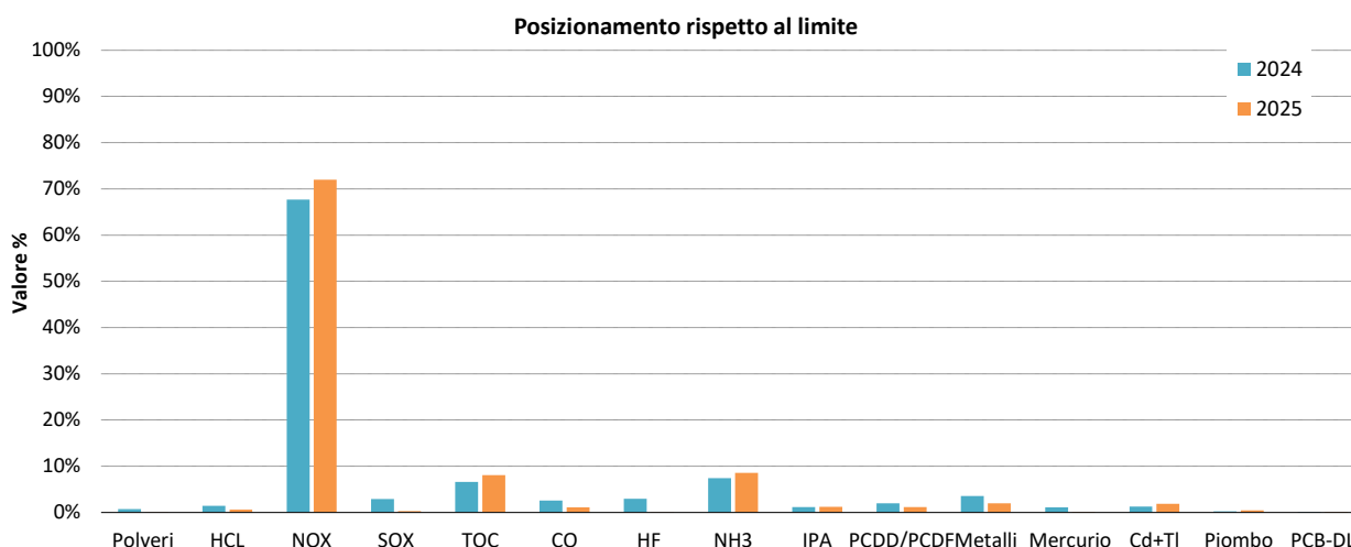
Figura 38 Andamento dell'indicatore "Posizionamento rispetto al limite" (E3)
