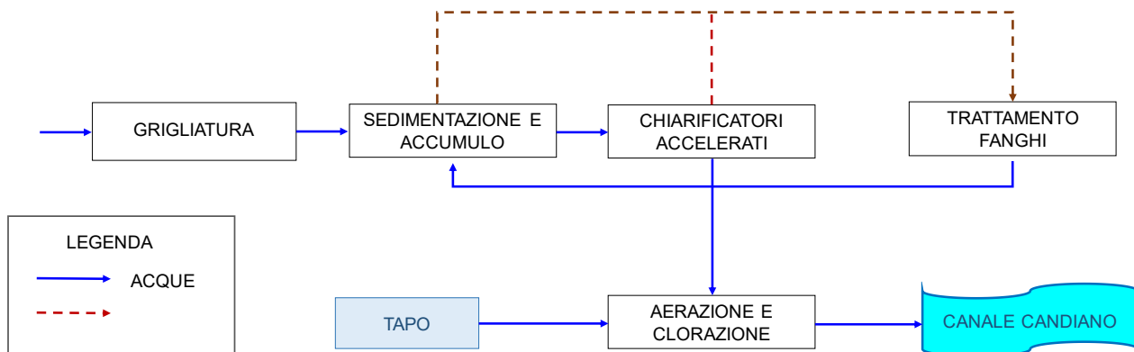
Figura 17 Ciclo produttivo (TAPI)
