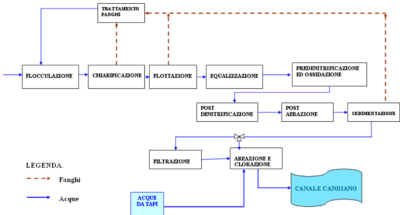
Figura 13 Ciclo produttivo (TAPO)
