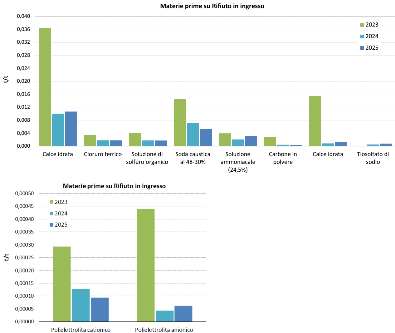
Figura 44 Andamento dell'indicatore "Fattore di utilizzo reagenti" (F3)
