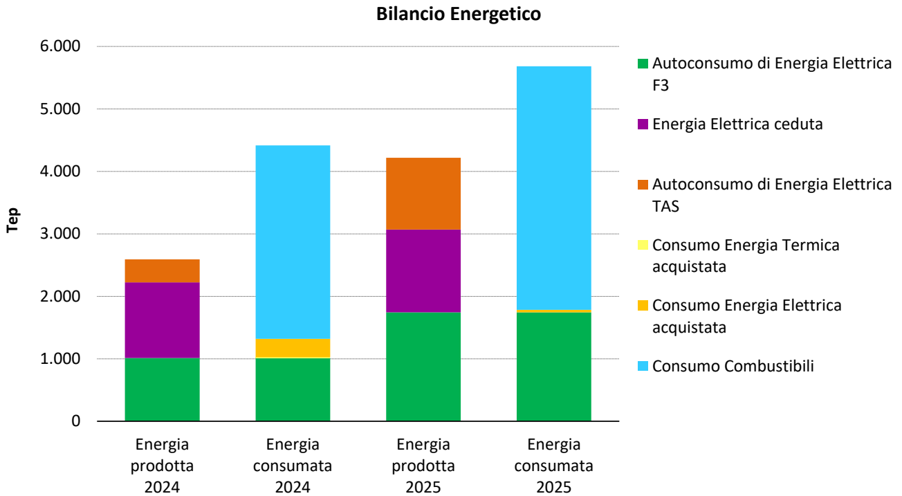
Figura 22 Bilancio energetico del termovalorizzatore (F3)
