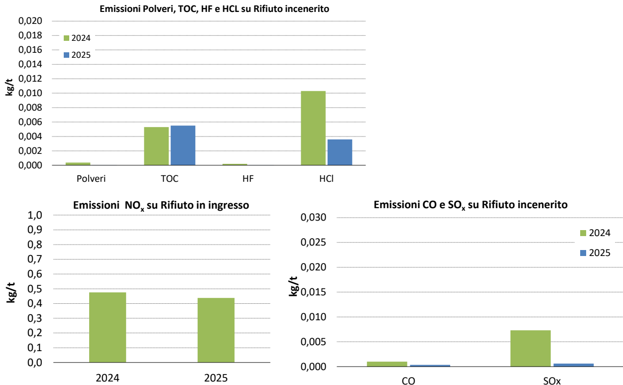
Figura 39 Andamento dell'indicatore "Fattori di emissione specifici" (E3)
