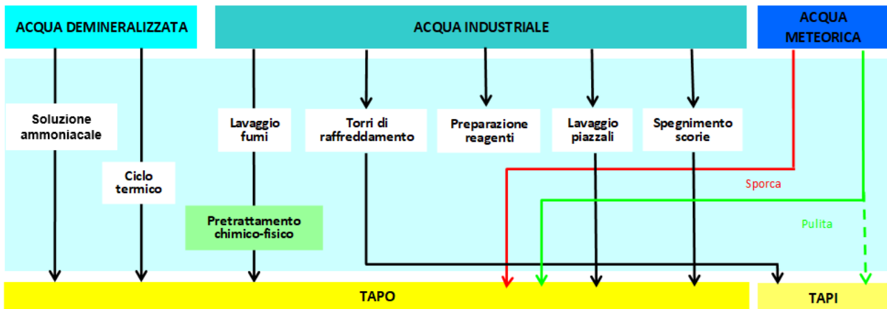
Figura 28 Ciclo idrico - F3
