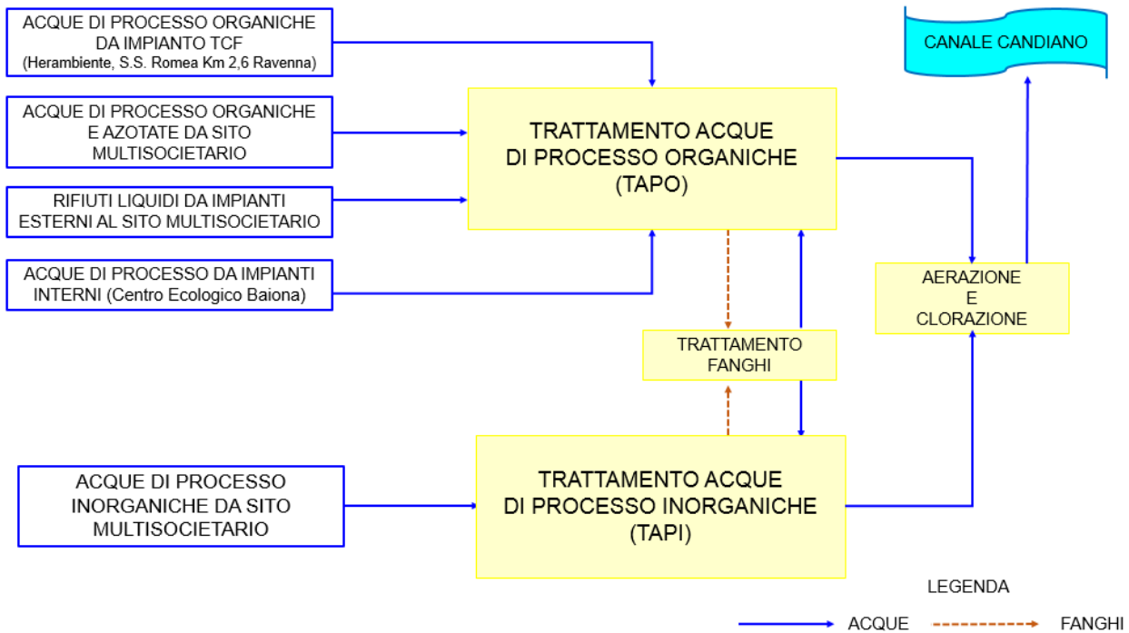
Figura 12 Ciclo produttivo (TAS)
