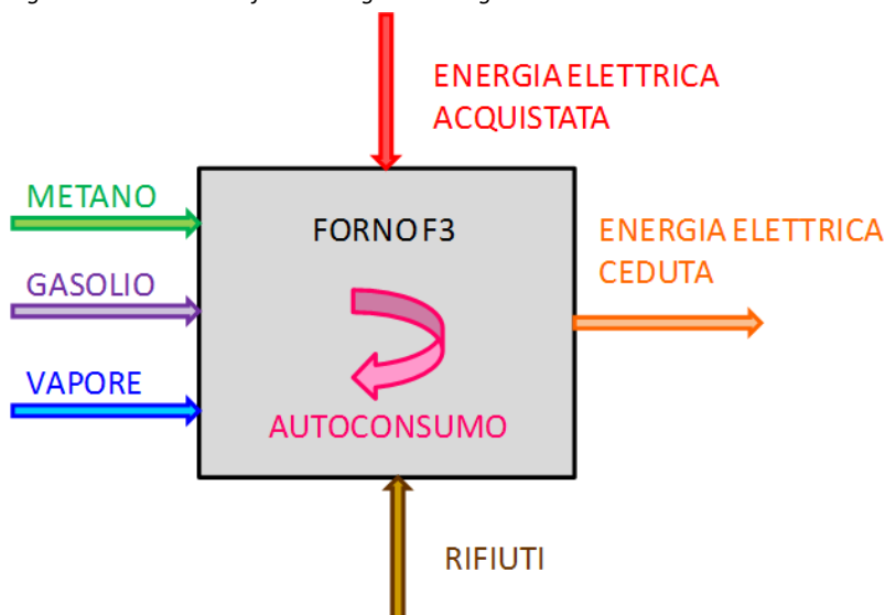
Figura 21 Schema dei flussi energetici in ingresso e in uscita nel Forno F3
