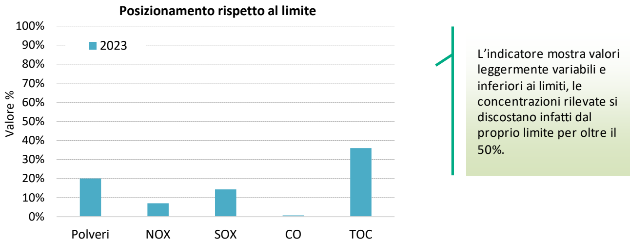
Figura 42 Andamento dell'indicatore "Posizionamento rispetto al Limite" (E4)
