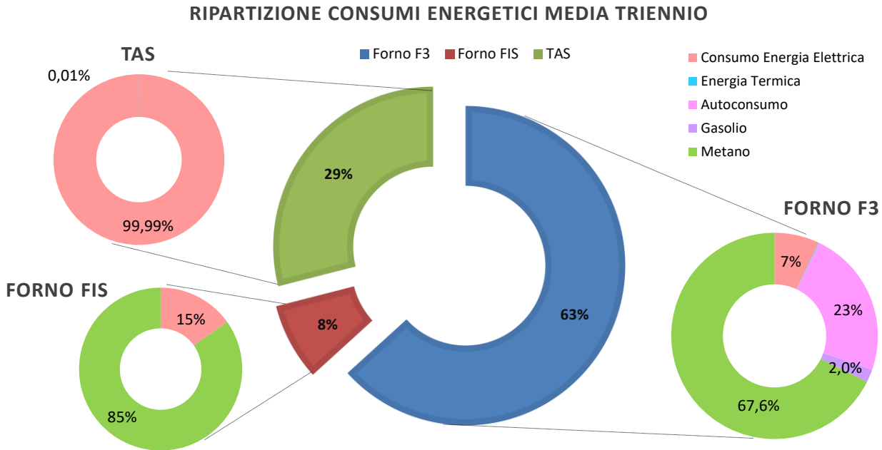
Figura 20 Ripartizione dei consumi energetici del sito (media 2023 - 2025)
