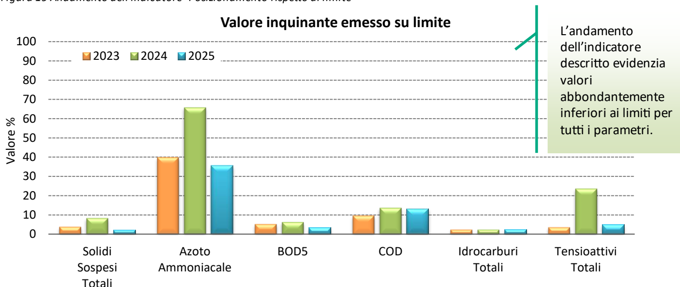
Figura 19 Andamento dell'indicatore "Posizionamento rispetto al limite"
