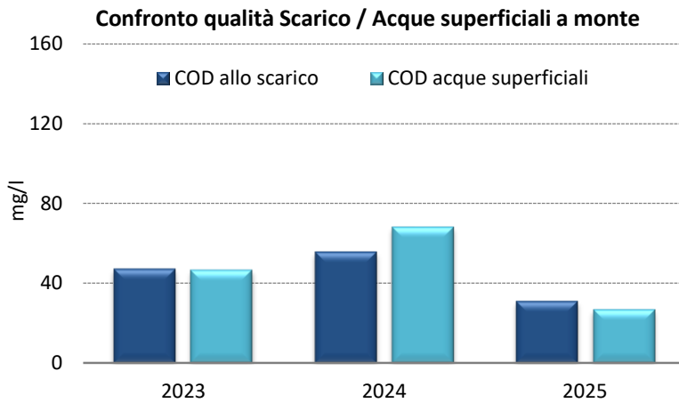
Figura 37 Confronto COD Scolo Tomba e media scarico (S5) – Media annua
