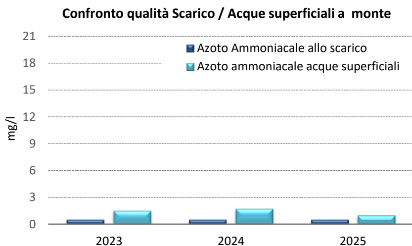
Figura 36 Confronto Azoto ammoniacale Scolo Tomba e media scarico (S5) – Media annua
