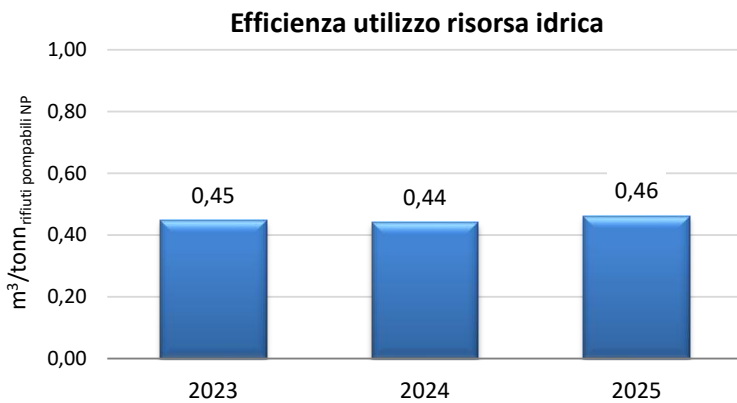
Figura 31 Andamento dell'indicatore "Efficienza di utilizzo della risorsa idrica"
