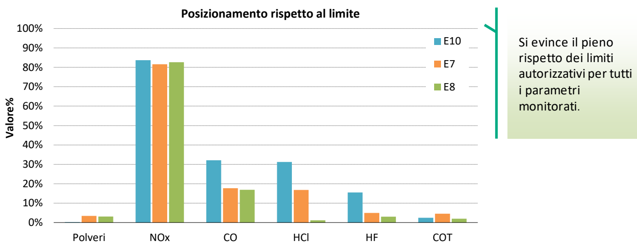
Figura 39 Andamento temporale dell'indicatore "Posizionamento rispetto al limite" (E10, E7, E8)
