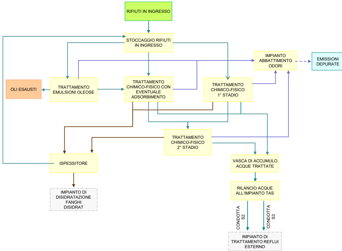
Figura 13 Ciclo produttivo dell'impianto di trattamento chimico-fisico (TCF)
