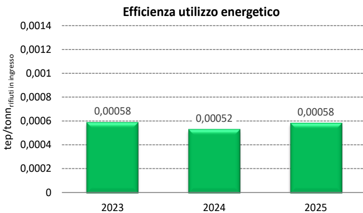
Figura 25 Andamento dell'indicatore "Efficienza di utilizzo energetico"
