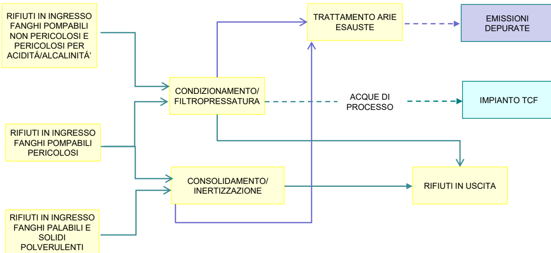
Figura 19 Ciclo produttivo impianto Disidrat
