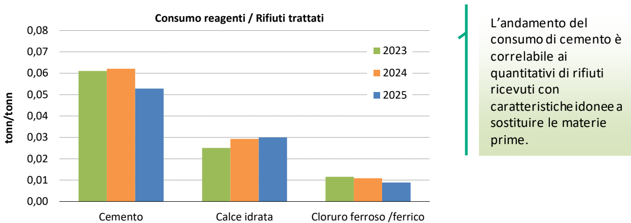
Figura 44 Andamento dell’indicatore “Consumo reagenti su rifiuti trattati”
