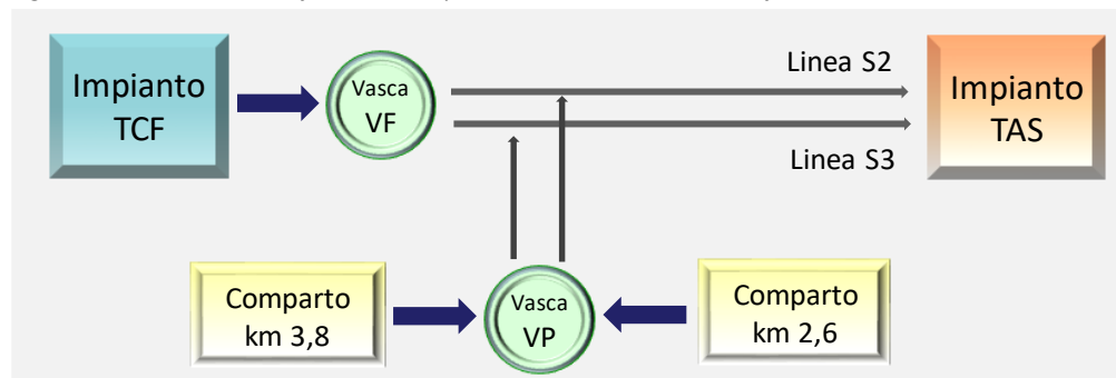
Figura 32 Schema sezione finale dell'impianto trattamento chimico-fisico
