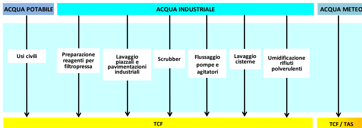
Figura 30 Ciclo idrico dell'impianto Disidrat
