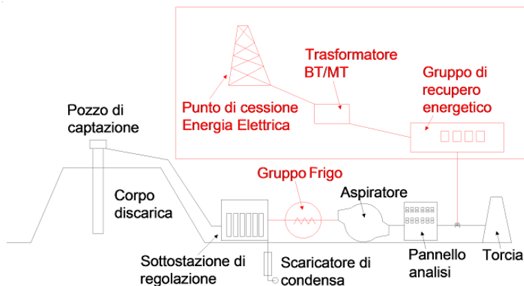
Figura 11 Schema del recupero energetico
