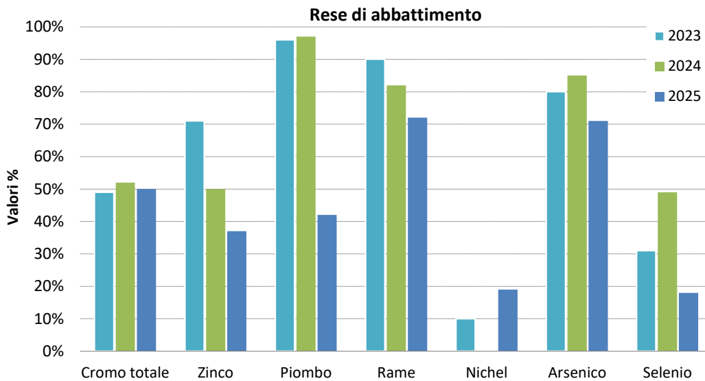
Figura 34 Andamento dell'indicatore "Efficienza di abbattimento" (TCF)
