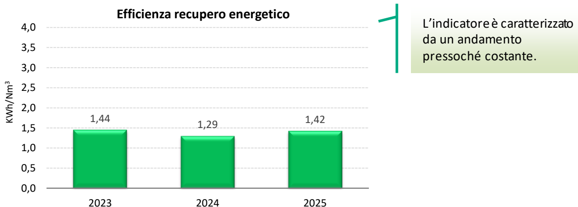
Figura 24 Andamento dell'indicatore "Efficienza di recupero energetico"
