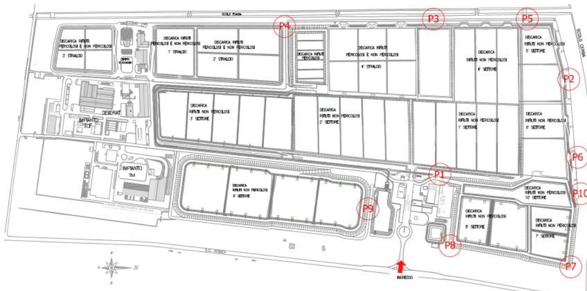
Figura 40 Planimetria dei punti di monitoraggio delle emissioni diffuse
