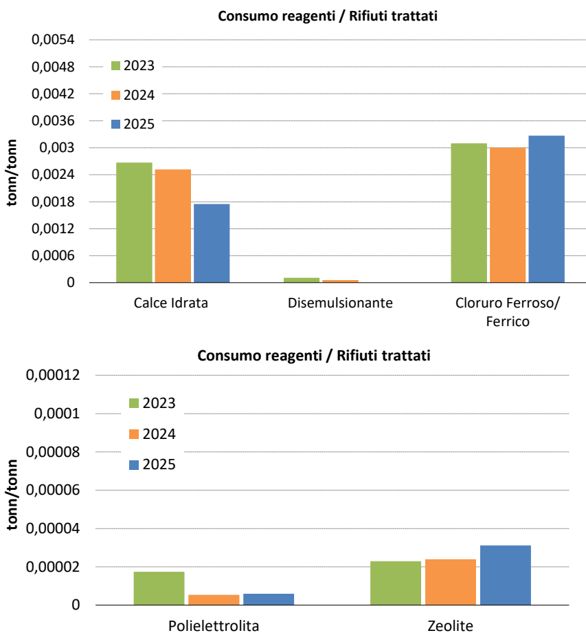
Figura 43 Andamento dell'indicatore "Fattore di utilizzo dei reagenti"
