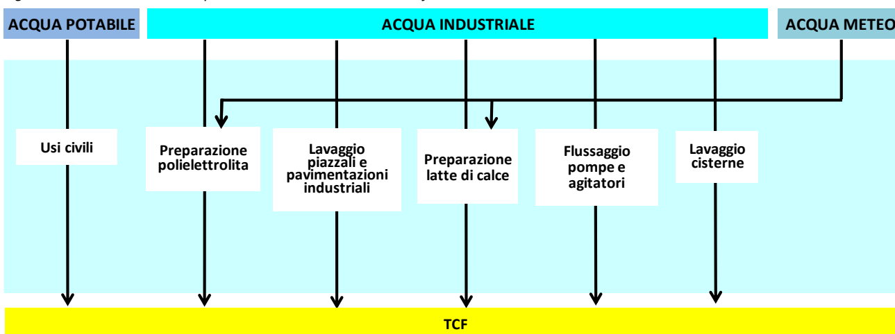
Figura 28 Ciclo idrico dell'impianto di trattamento chimico-fisico
