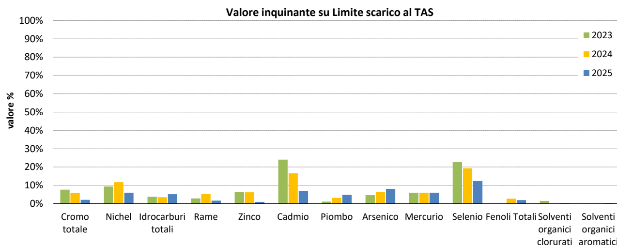
Figura 33 Andamento dell'indicatore "Posizionamento rispetto al limite" – Scarico verso il TAS
