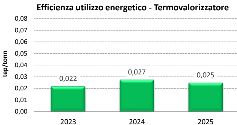
Figura 19 Andamento dell'indicatore "Efficienza di utilizzo energetico"
