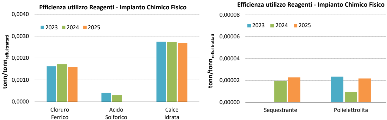
Figura 40 Andamento dell'indicatore "Fattore di utilizzo reagenti"
