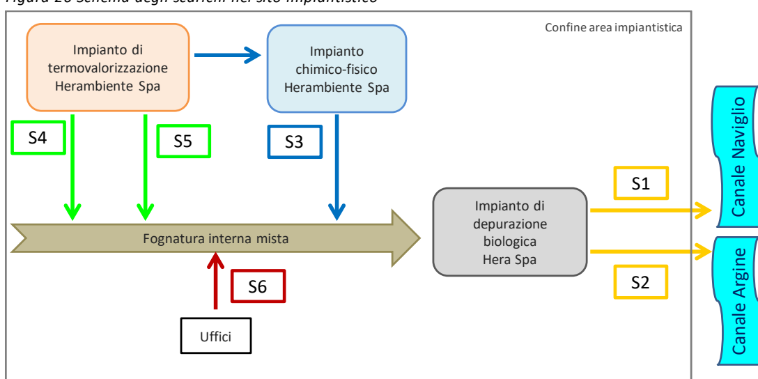
Figura 26 Schema degli scarichi nel sito impiantistico
