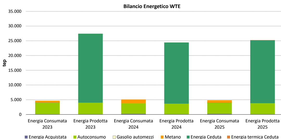
Figura 17 Bilancio energetico del termovalorizzatore
