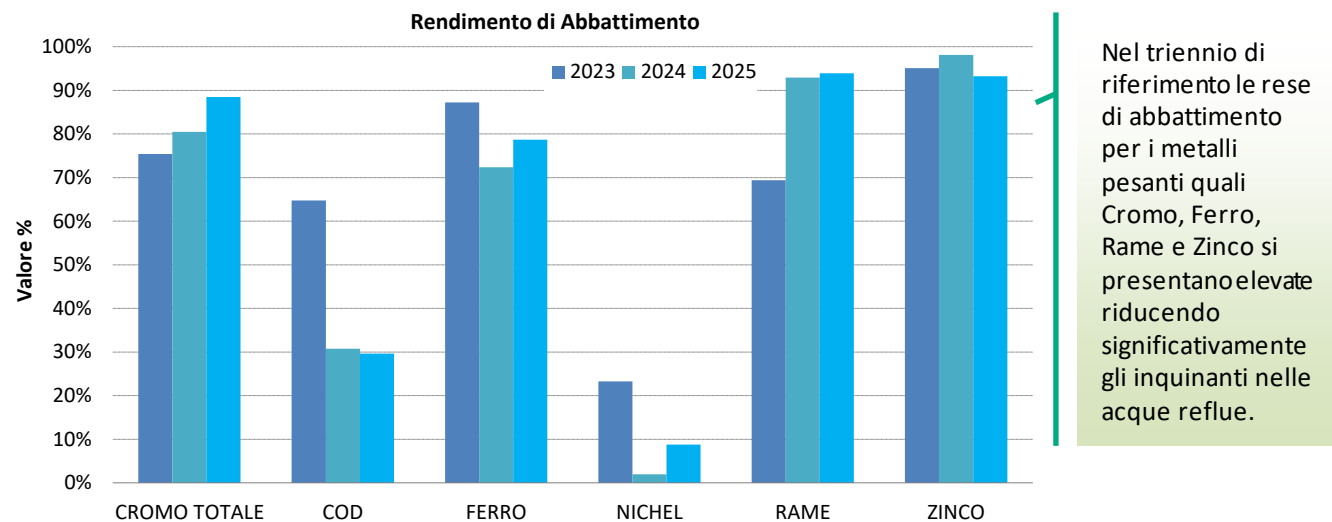
Figura 28 Rendimenti di abbattimento
