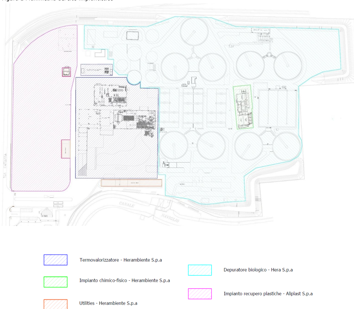
Figura 1 Planimetria del sito impiantistico
