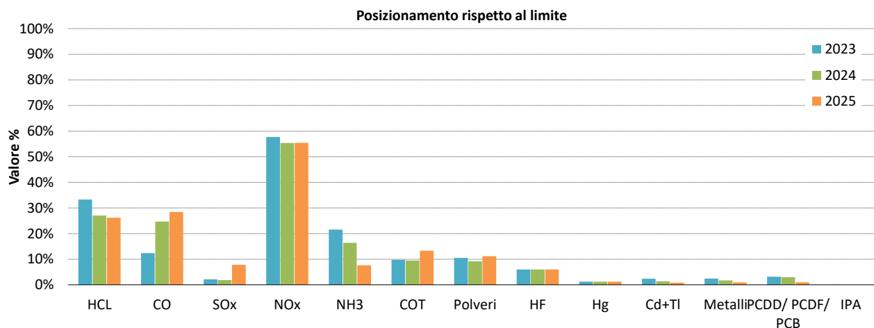
Figura 32 Andamento dell'indicatore "Posizionamento rispetto al limite" – Linea 4
