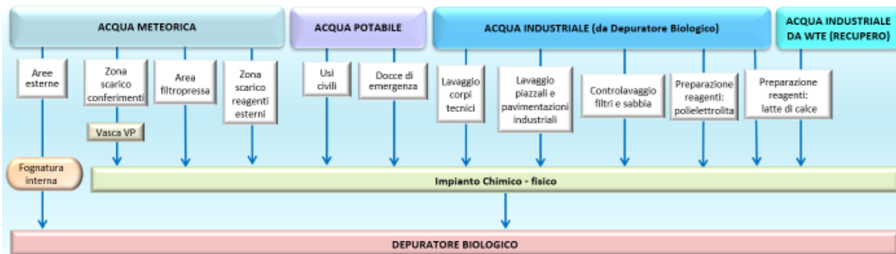
Figura 24 Ciclo idrico dell'impianto chimico-fisico
