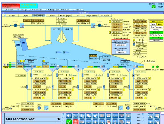
Figura 10 Schermata software di controllo parametri della combustione
