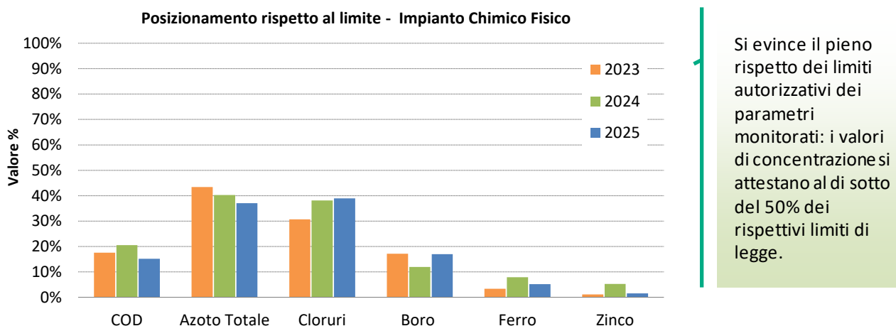
Figura 27 Andamento dell'indicatore "Posizionamento rispetto al limite" (S3)
