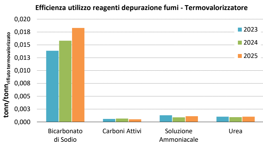
Figura 39 Andamento dell'indicatore "Fattore di utilizzo reagenti"
