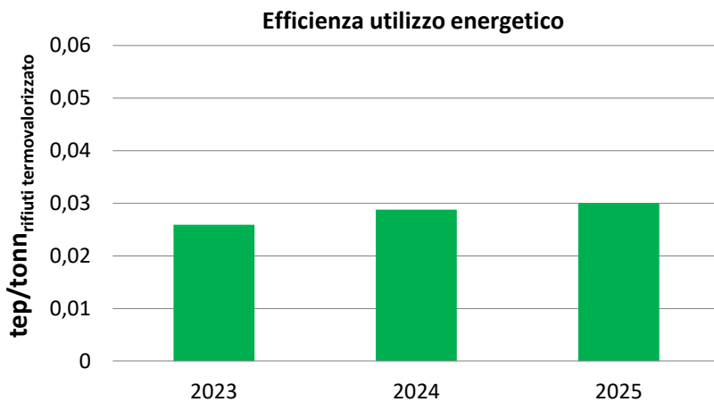
Figura 25 Andamento dell'indicatore "Efficienza di utilizzo energetico"
