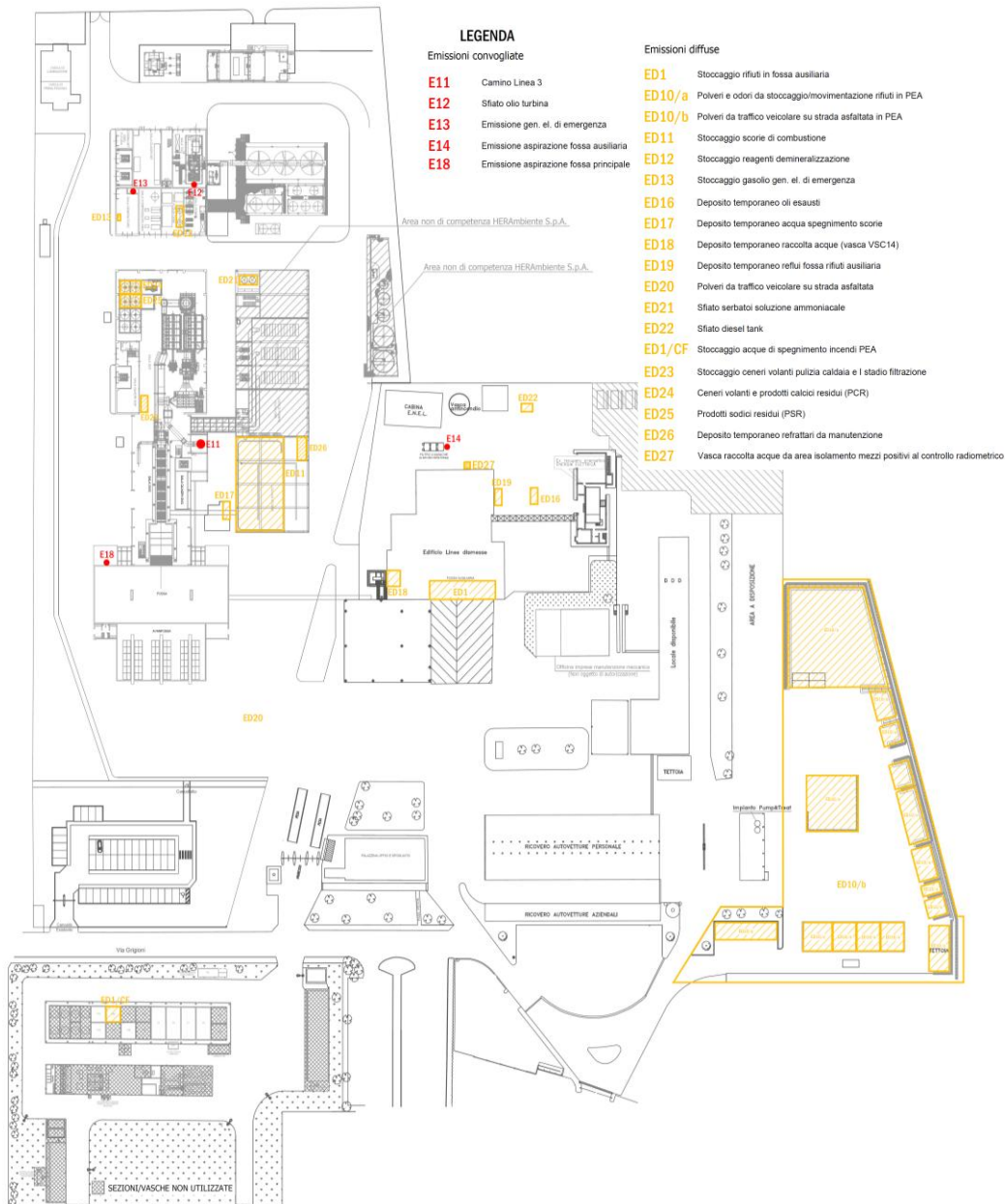
Figura 34 Planimetria delle emissioni del sito
