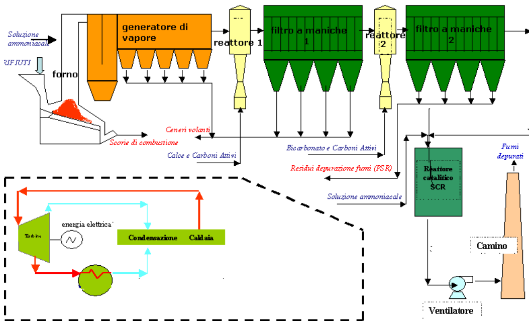
Figura 5 Ciclo produttivo del termovalorizzatore
