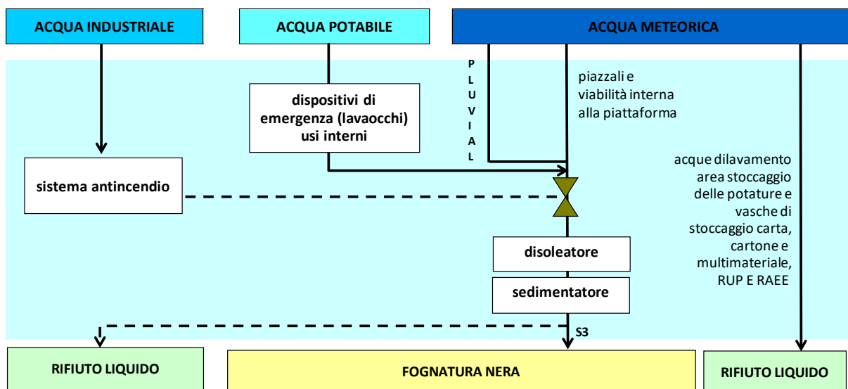
Figura 29 Ciclo idrico della piattaforma ecologica
