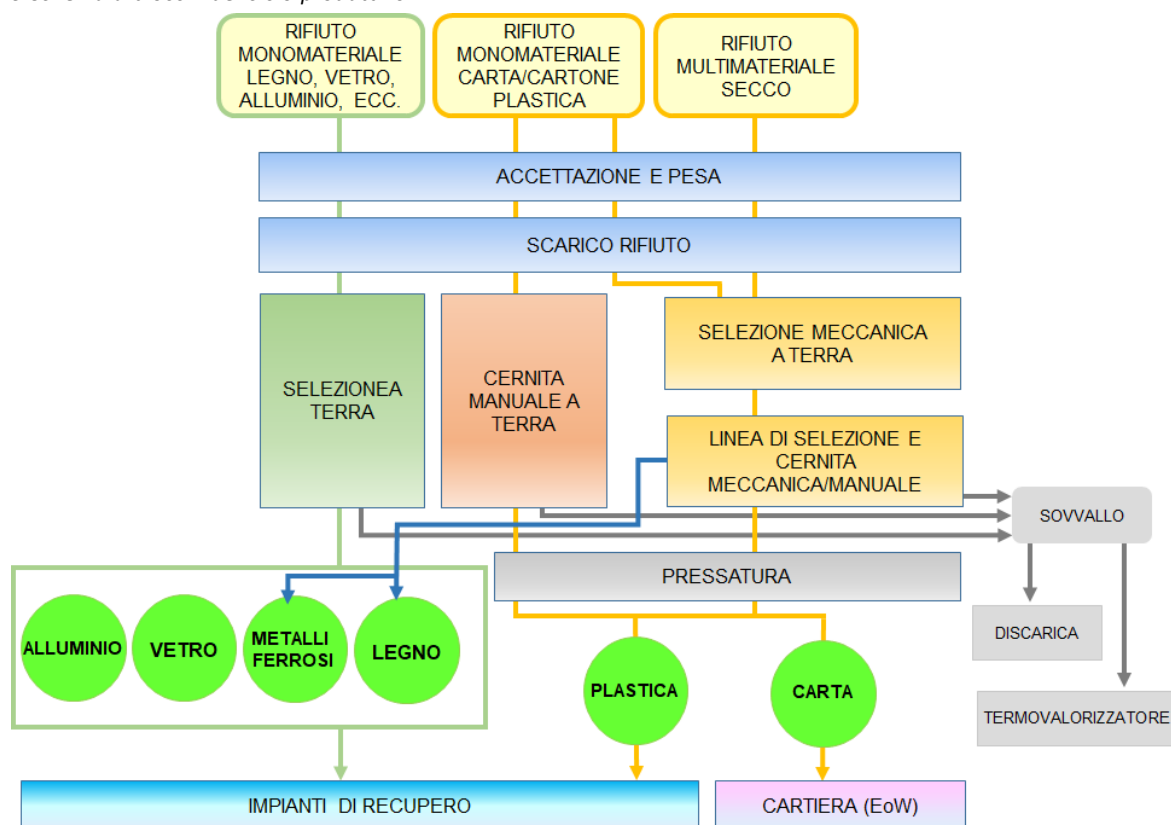
Figura 5 Schema a blocchi del ciclo produttivo
