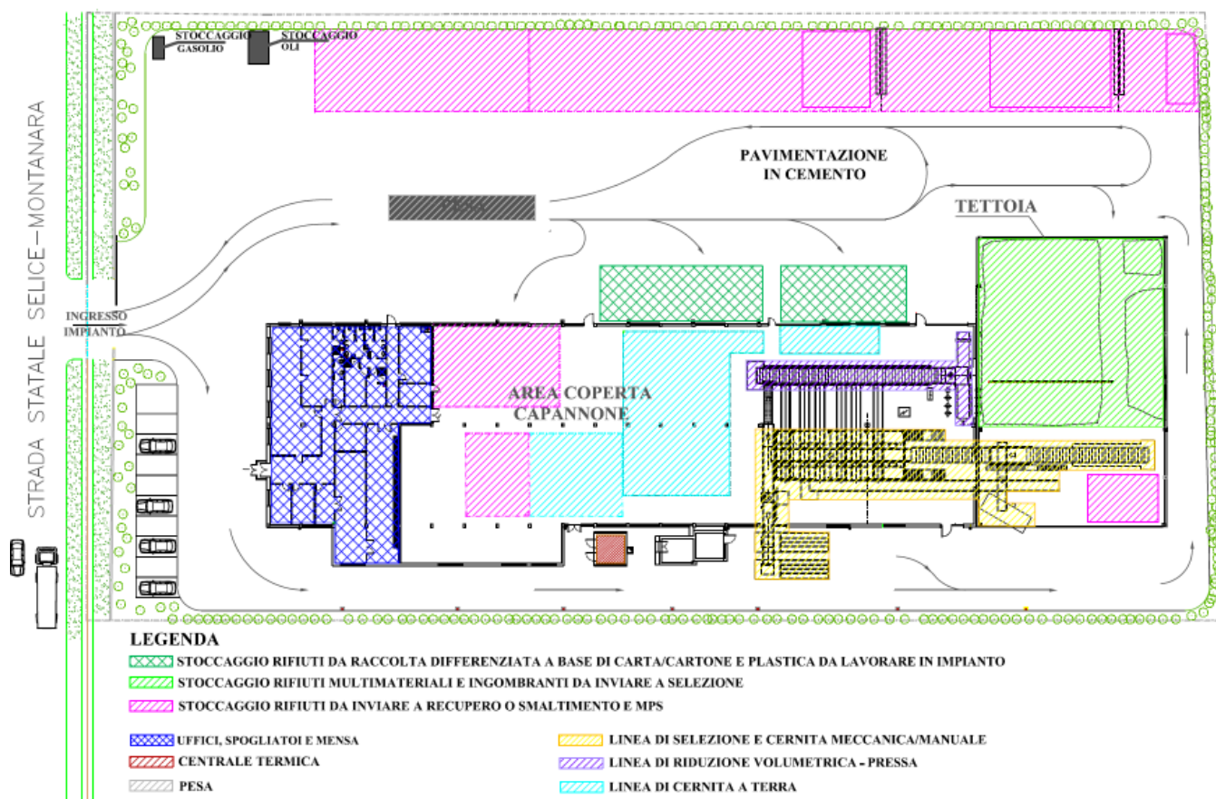
Figura 2 Planimetria del sito
