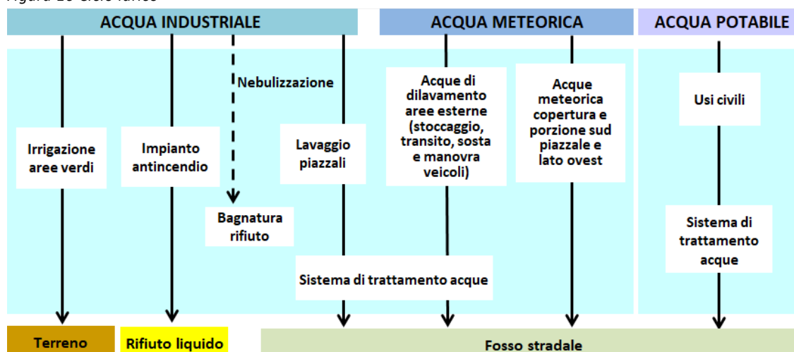
Figura 16 Ciclo idrico
