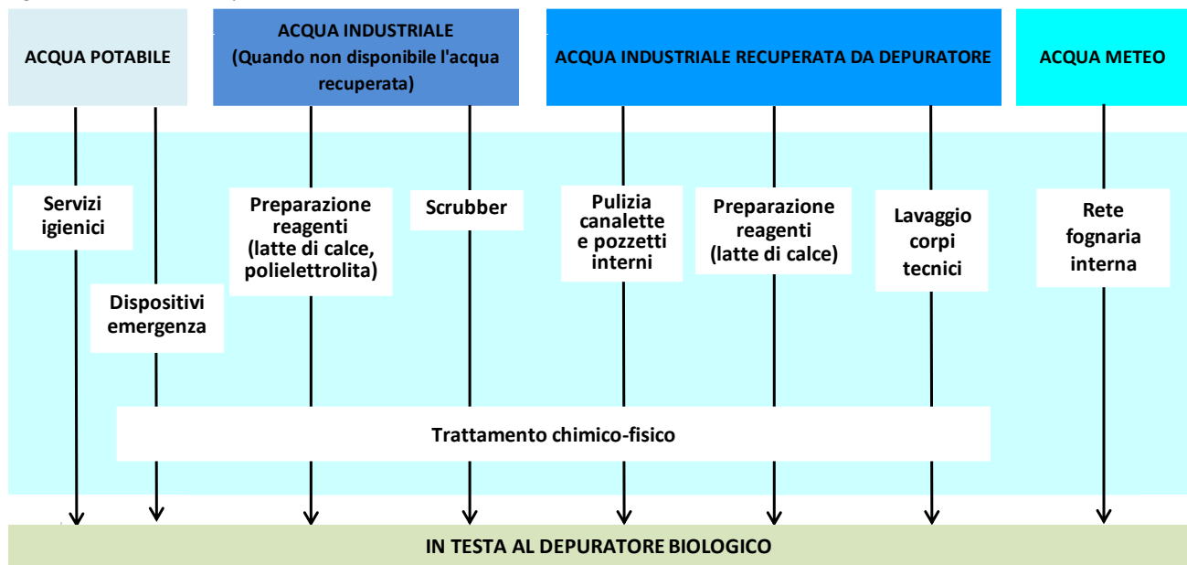
Figura 14 Ciclo idrico Impianto
