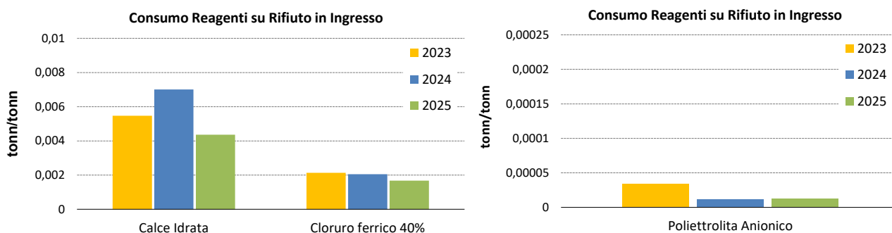
Figura 20 Andamento dell'indicatore "Fattore di utilizzo reagenti"
