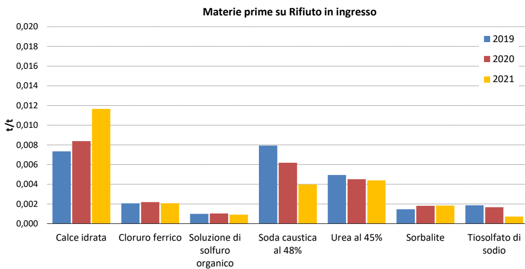
Figura 45 Andamento dell'indicatore "Fattore di utilizzo reagenti" (F3)
