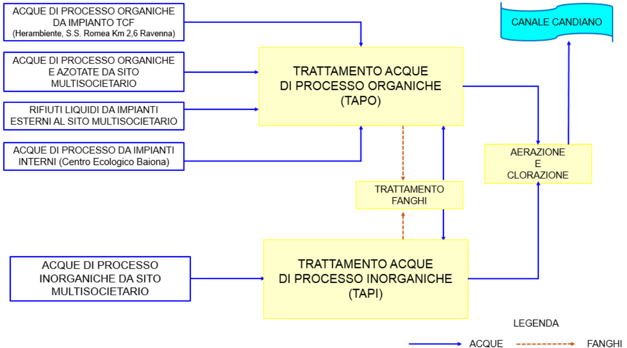
Figura 13 Ciclo produttivo (TAS)
