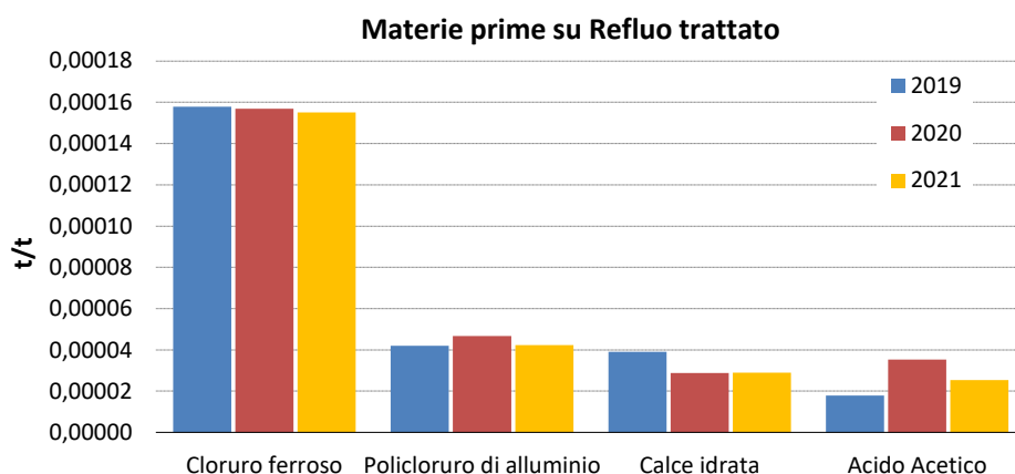
Figura 46 Andamento dell'indicatore "Fattore di utilizzo reagenti" (TAS)
