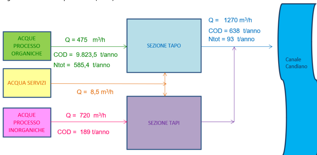
Figura 37 Bilancio impianto TAS (2021)
