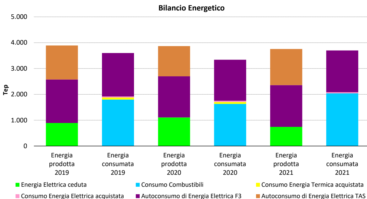
Figura 23 Bilancio energetico del termovalorizzatore (F3)
