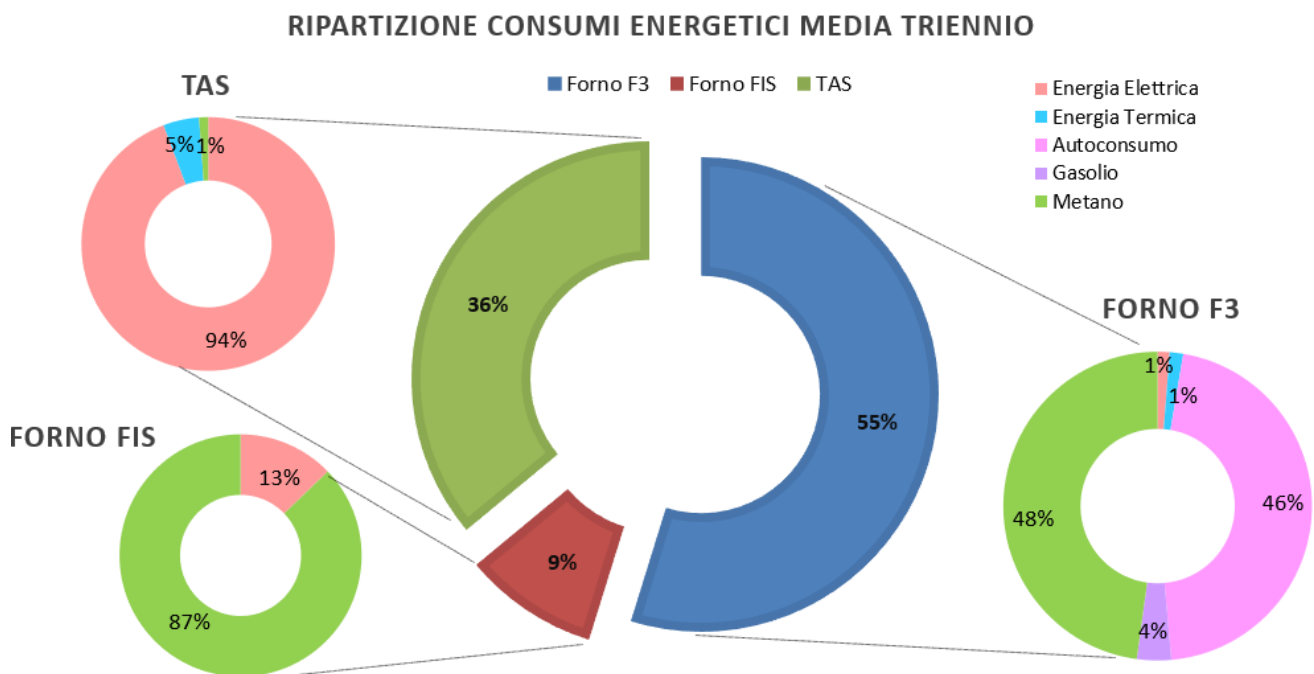
Figura 21 Ripartizione dei consumi energetici del sito (media 2019 - 2021)
