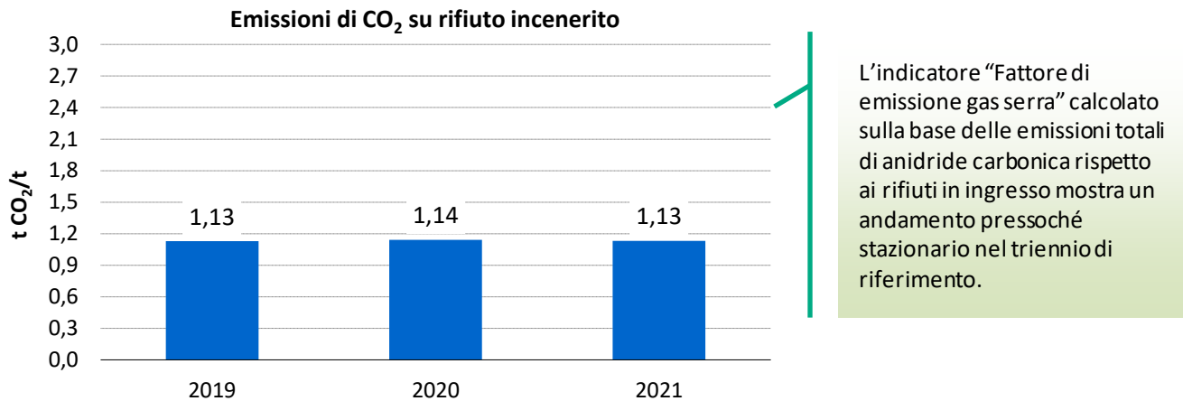
Figura 44 Andamento dell'indicatore "Fattore di emissione gas serra" (F3)
