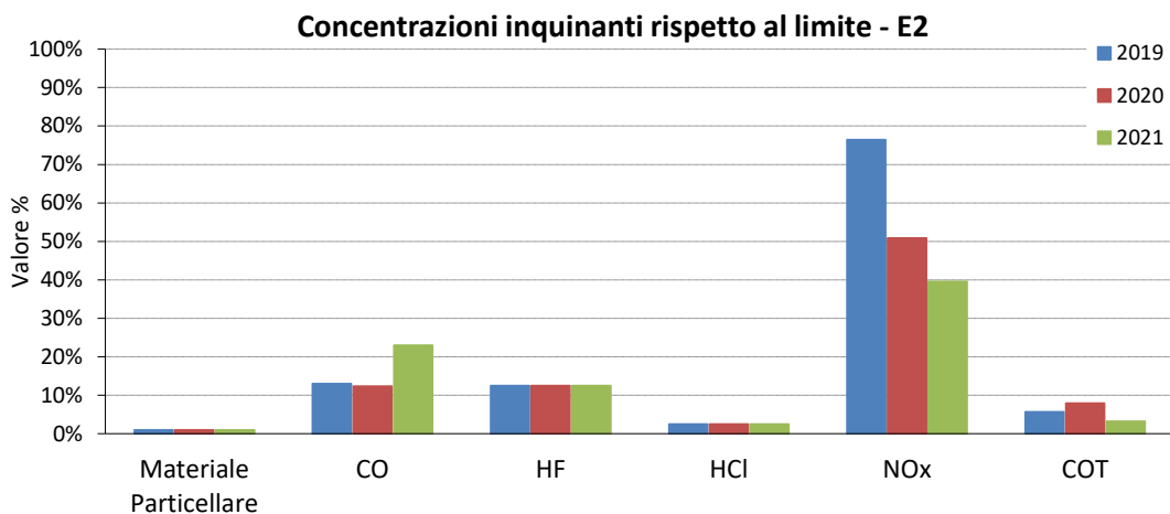
Figura 26 Andamento dell'indicatore "Posizionamento rispetto al limite" (E2)
