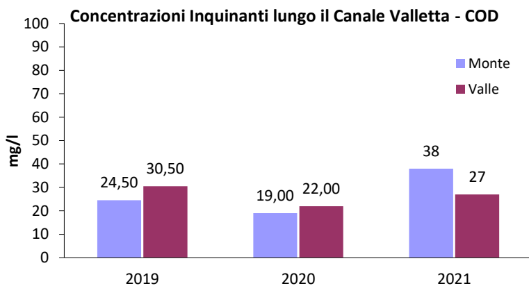
Figura 20 Confronto COD a monte e a valle del sito
