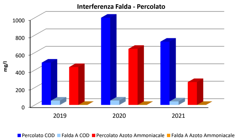
Figura 24 Confronto tra gli andamenti dei markers nel percolato e nella falda A di primo livello
