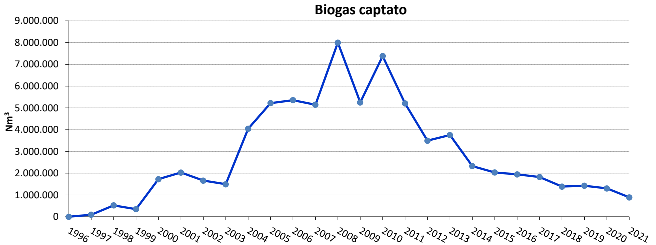
Figura 12 Quantitativi di biogas estratto durante il ciclo di vita della discarica
