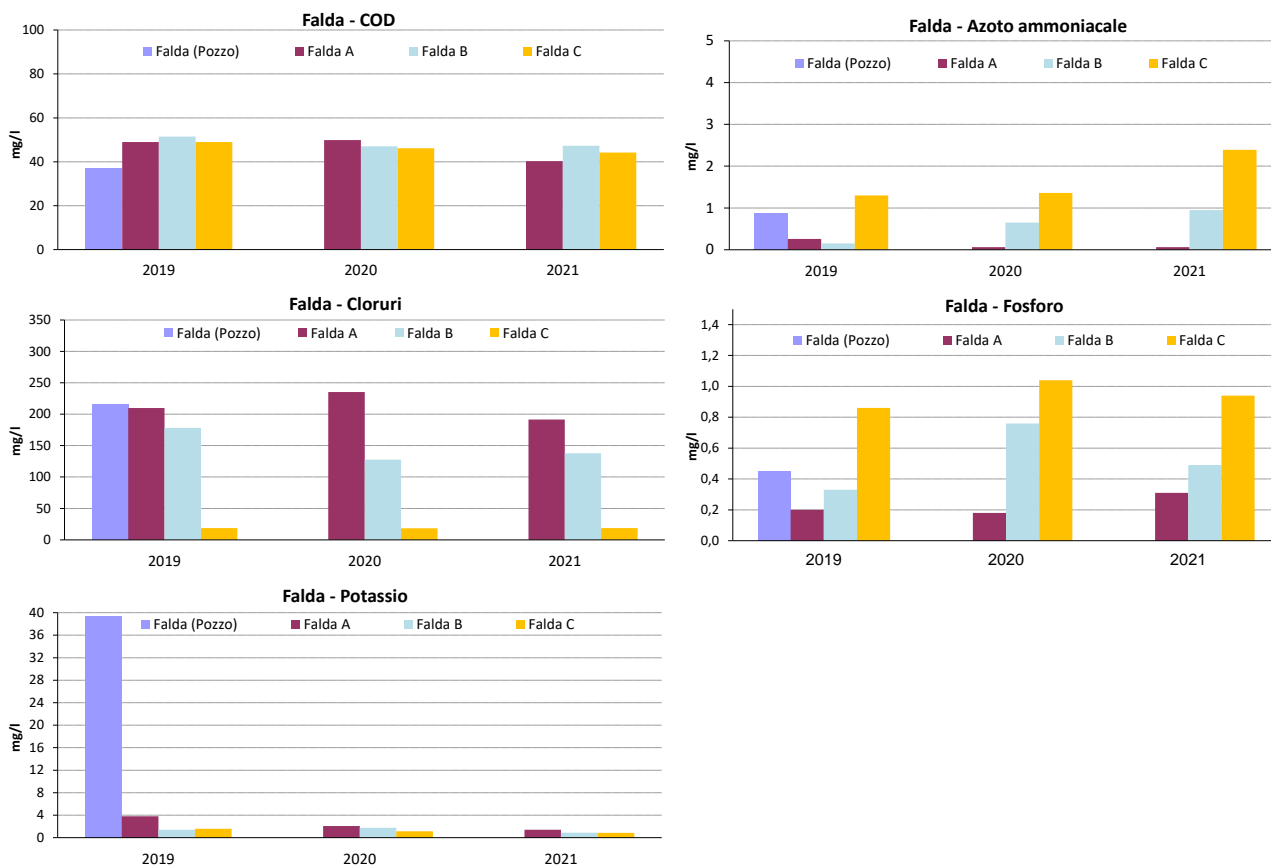
Figura 23 Andamento del COD e dei markers per le acque di falda
