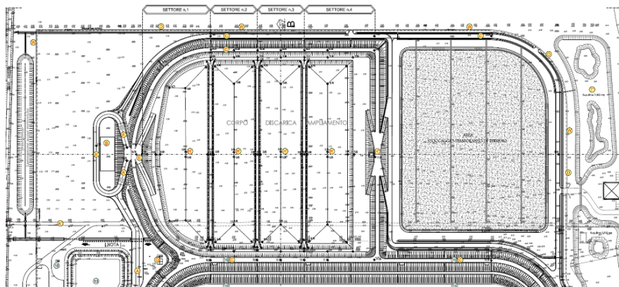
Figura 4 Particolare da progetto nuova discarica
