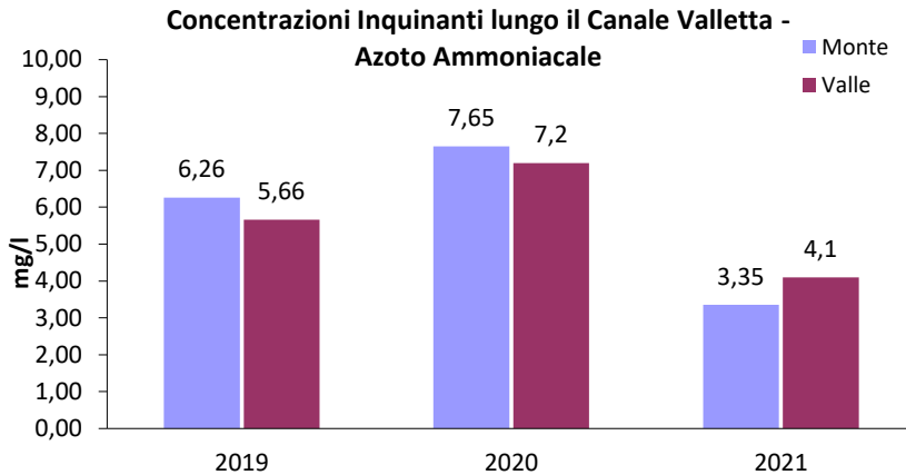
Figura 19 Confronto Azoto ammoniacale a monte e a valle del sito
