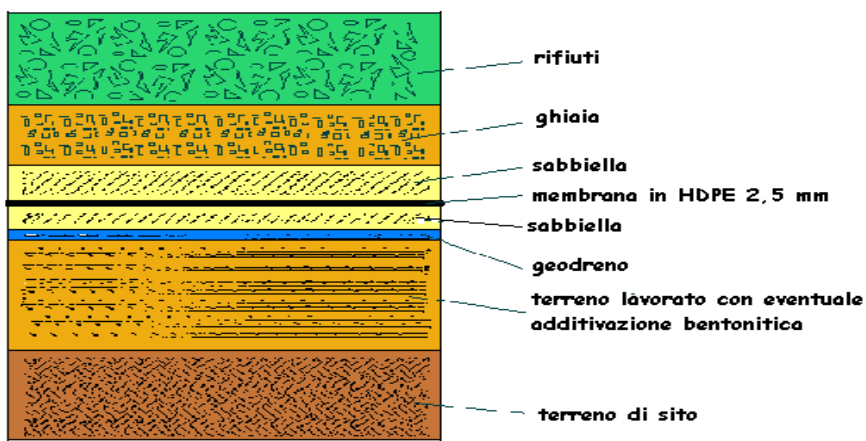
Figura 21 Struttura del fondo della discarica
