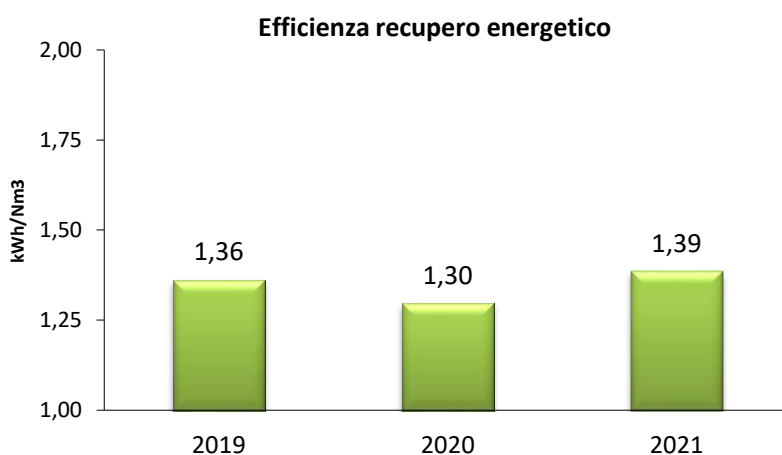
Figura 15 Andamento dell'indicatore "Efficienza di Recupero Energetico"
