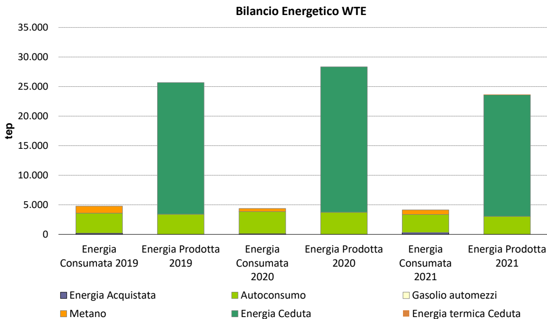
Figura 17 Bilancio energetico del termovalorizzatore
