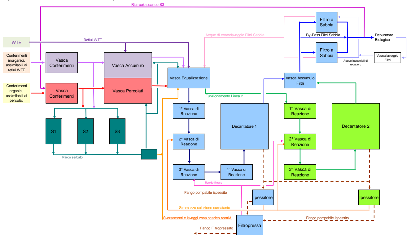
Figura 13 Schema a blocchi del ciclo produttivo
