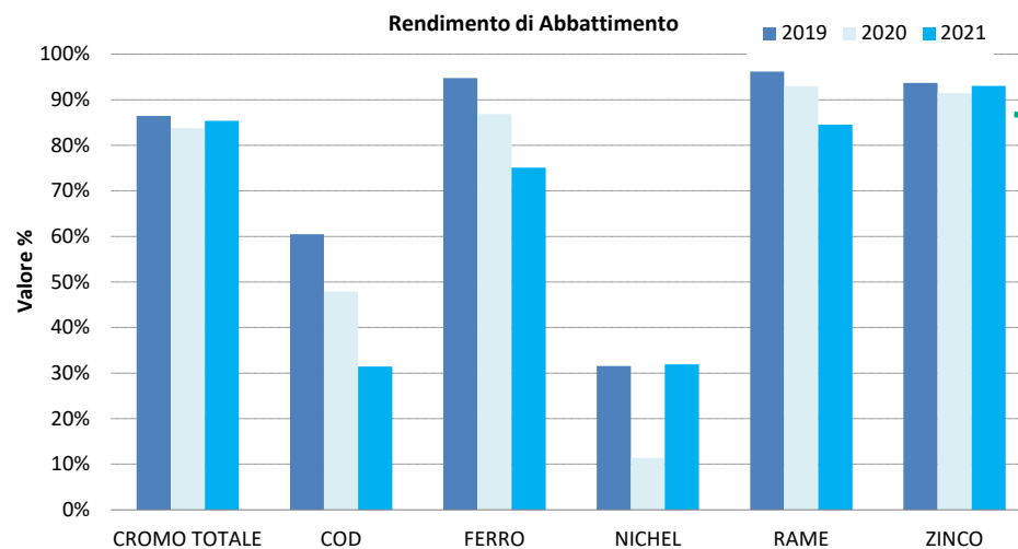
Figura 28 Rendimenti di abbattimento
