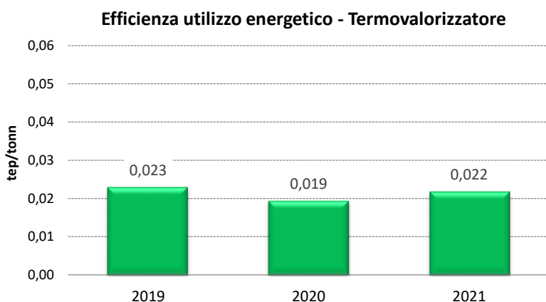
Figura 19 Andamento dell'indicatore "Efficienza di utilizzo energetico"
