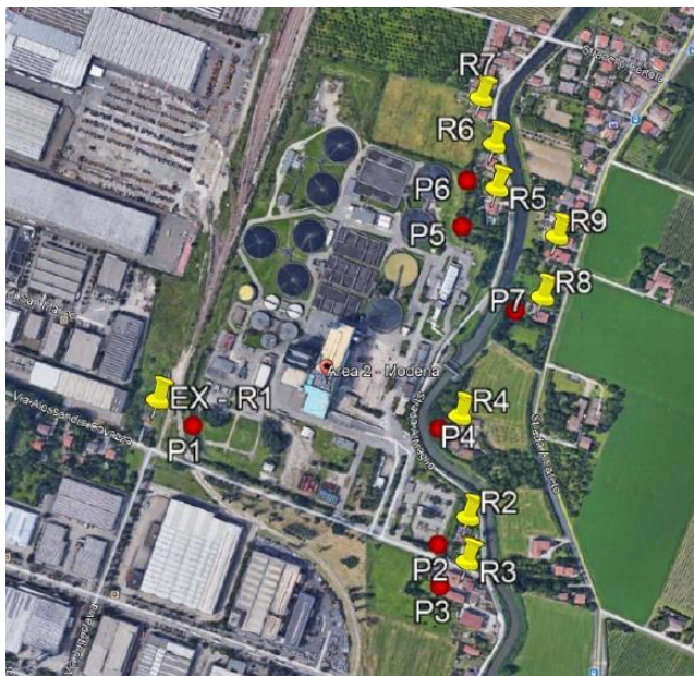
Figura 41 Localizzazione dei punti di campionamento fonometrico (P) e recettori (R)
