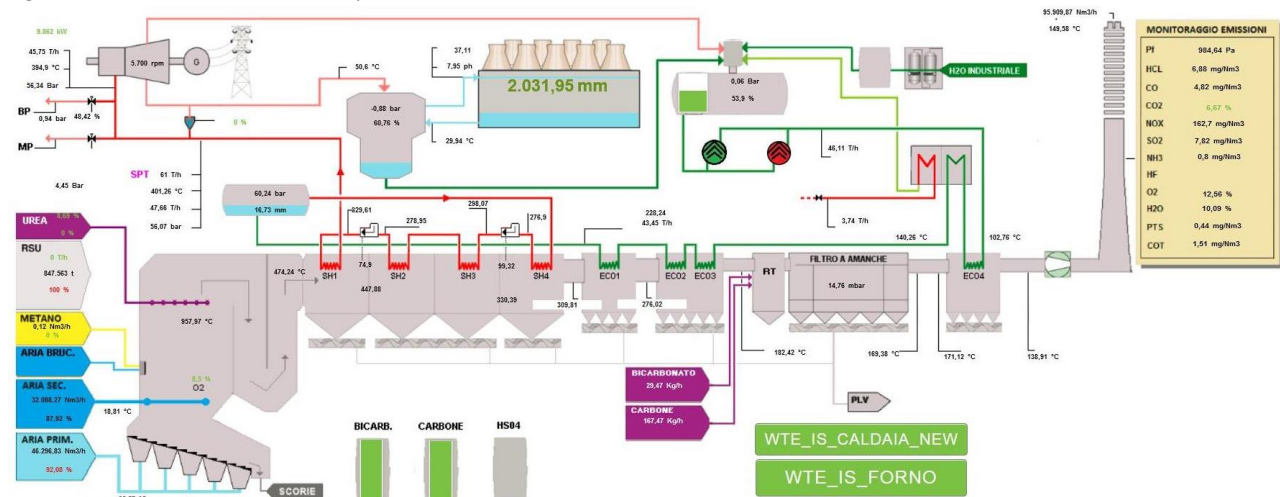
Figura 8 Schermata di controllo del processo
