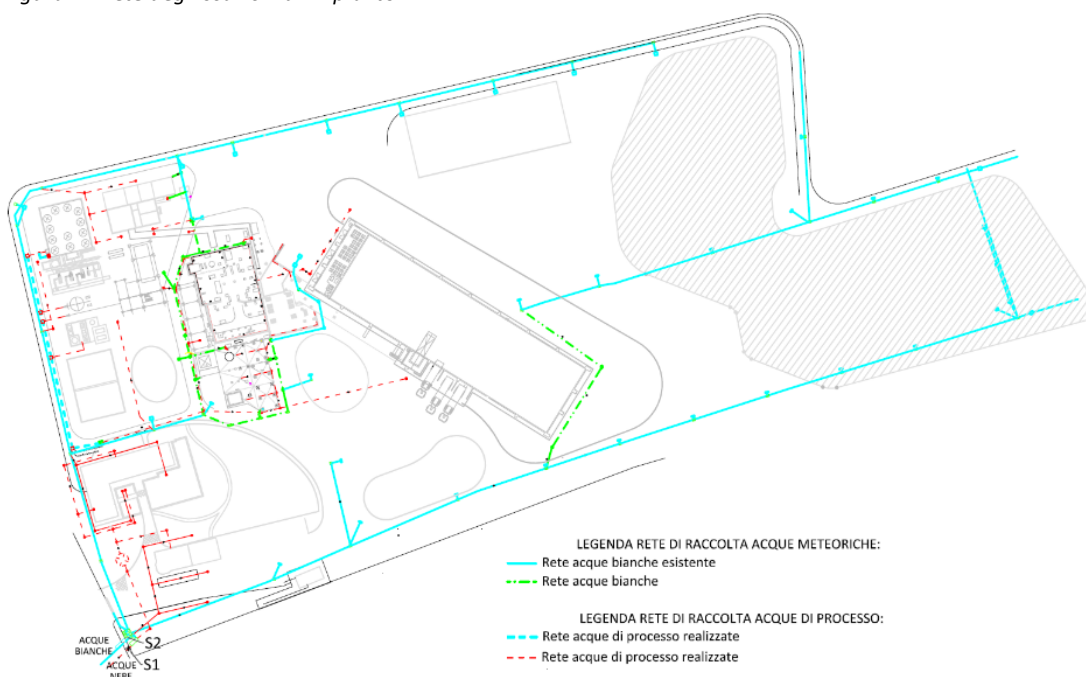
Figura 14 Rete degli scarichi di impianto
