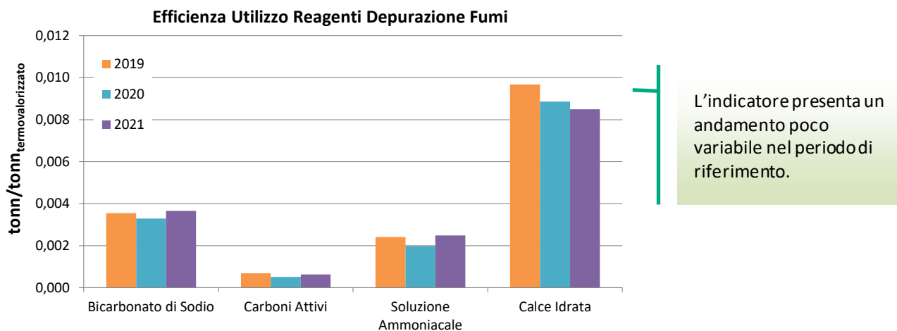
Figura 43 Andamento dell'indicatore "Fattore di utilizzo reagenti"
