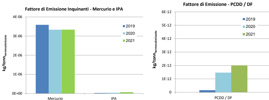
Figura 39 Andamento dell'indicatore "Fattori di Emissione Microinquinanti"
