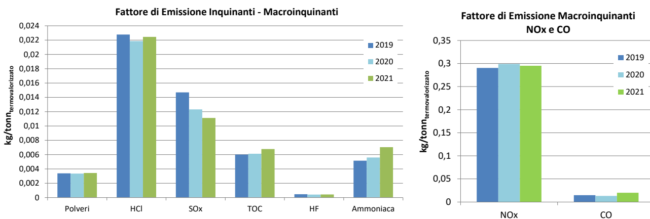
Figura 38 Andamento dell'indicatore "Fattori di Emissione Macroinquinanti"
