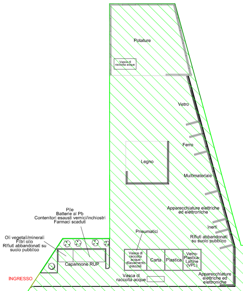
Figura 20 Organizzazione della piattaforma ecologica
