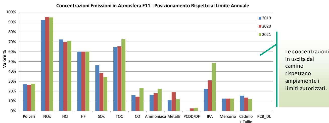
Figura 37 Andamento dell'indicatore "Posizionamento Rispetto al Limite"
