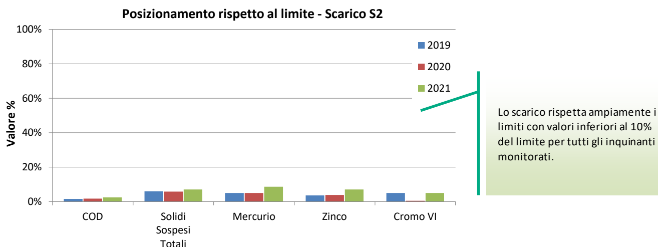
Figura 31 Andamento dell'indicatore "Posizionamento Rispetto al Limite" (S2)
