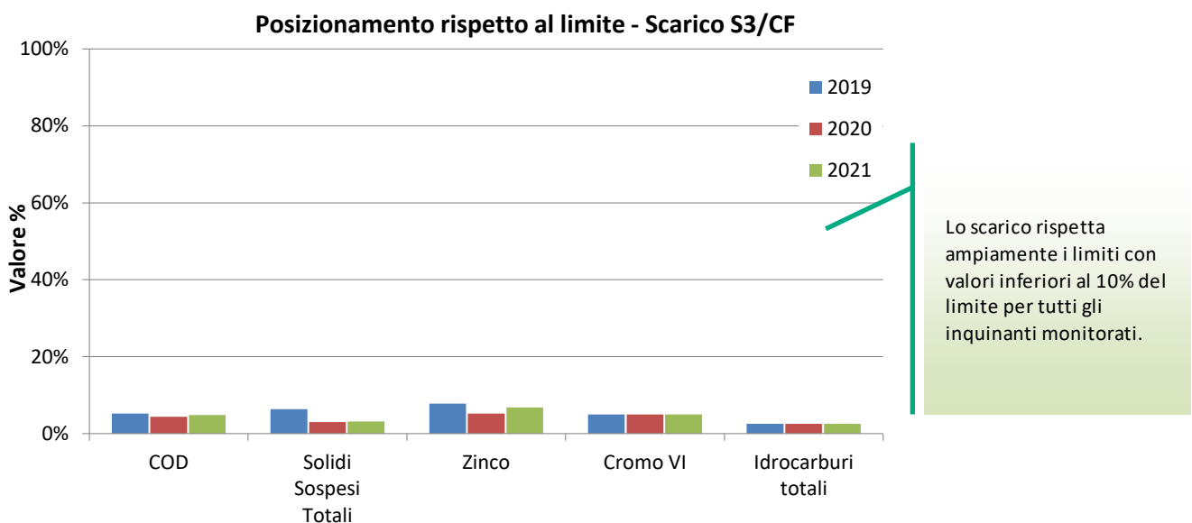
Figura 34 Andamento dell'indicatore "Posizionamento Rispetto al Limite" (S3/CF)
