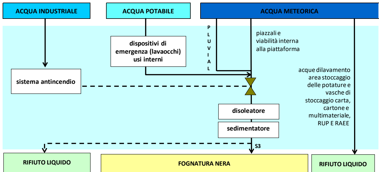
Figura 30 Ciclo idrico della piattaforma ecologica
