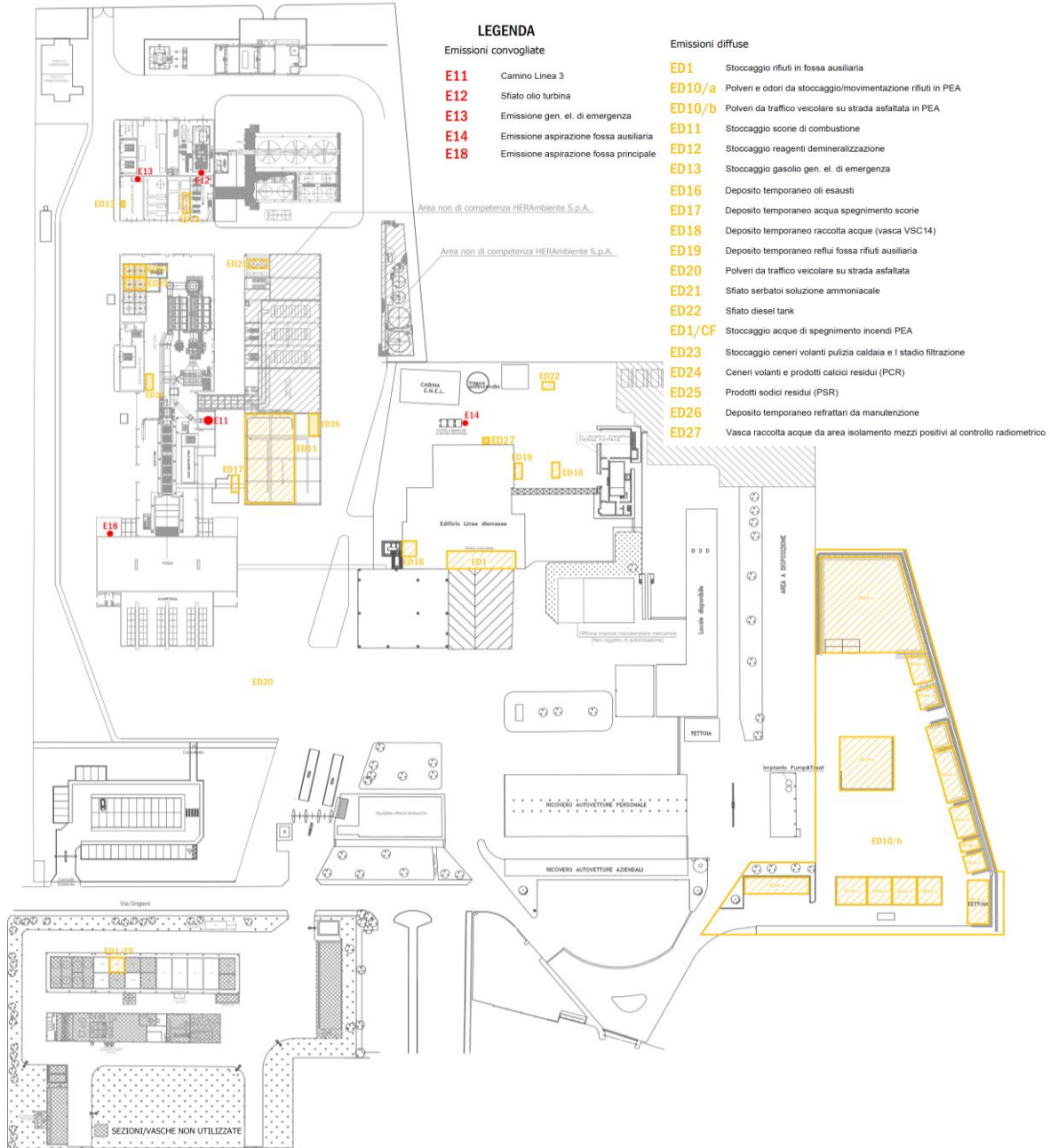
Figura 35 Planimetria delle emissioni del sito
