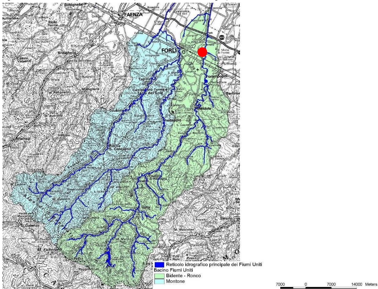
Figura 2 Reticolo idrografico dei Fiumi Uniti (Fonte: ARPAE Emilia-Romagna)
