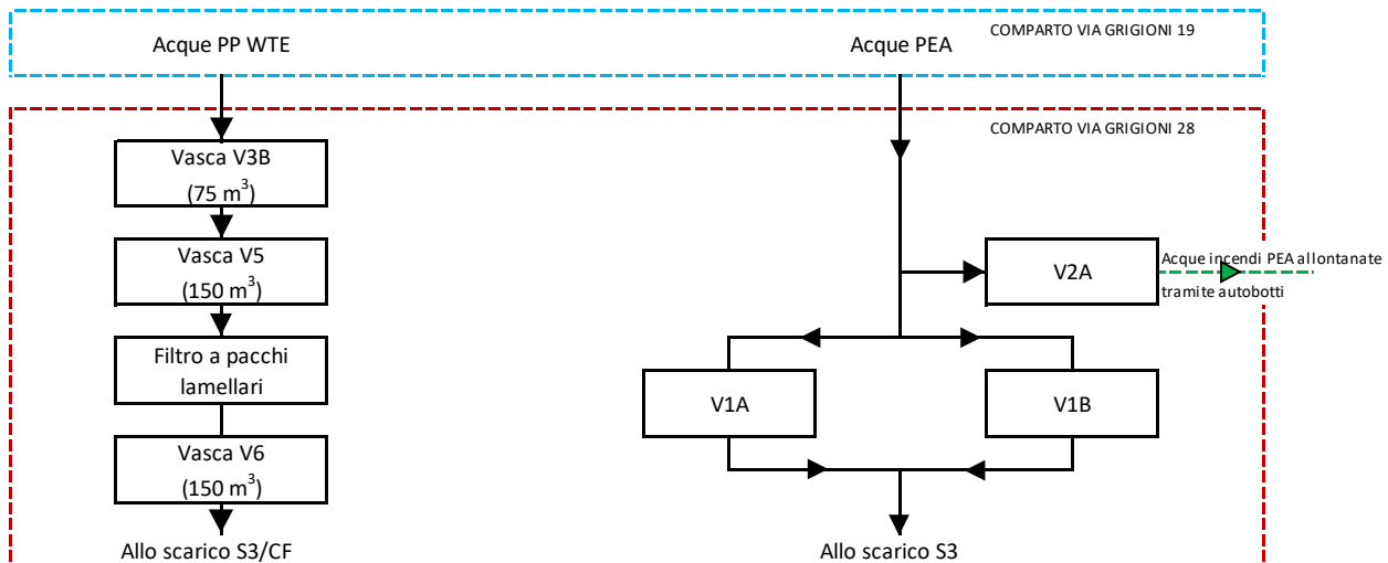
Figura 16 Schema a blocchi unità di trattamento chimico-fisico reflui
