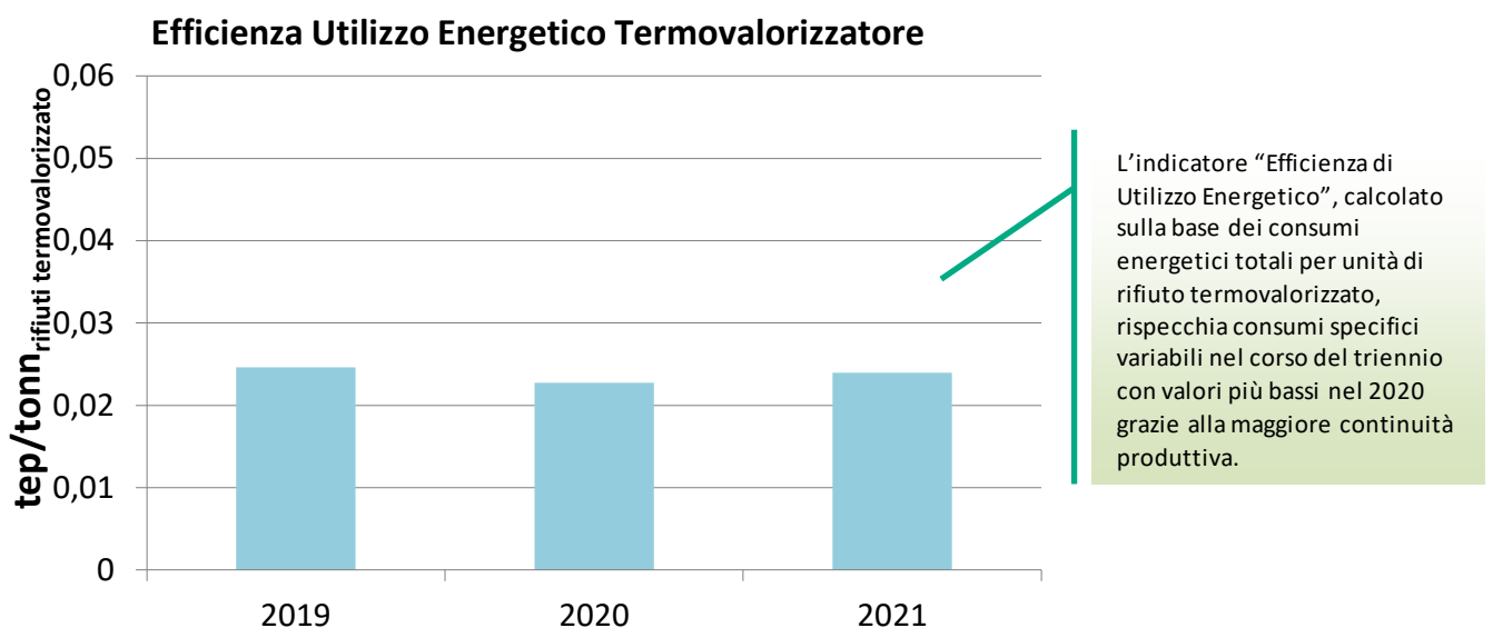
Figura 26 Andamento dell'indicatore "Efficienza di Utilizzo Energetico"
