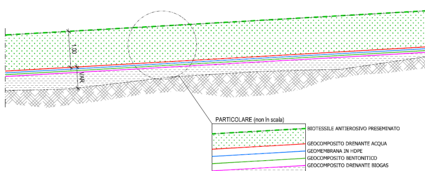
Figura 30 Particolare della copertura finale (piano sommitale)
