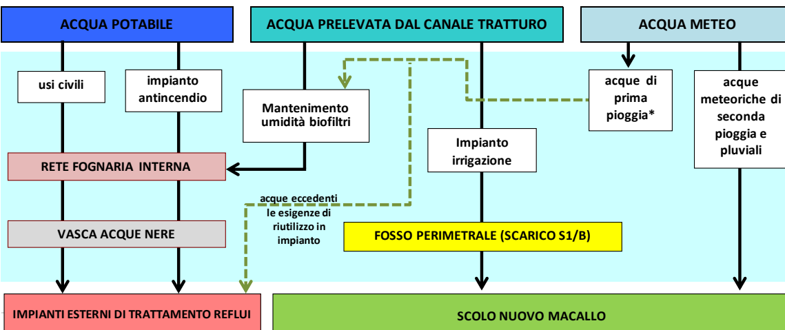
Figura 44 Ciclo idrico dell'impianto di compostaggio
