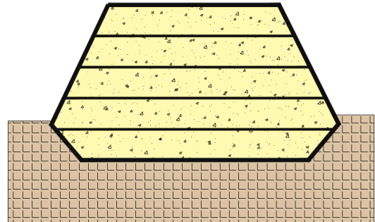
Figura 28 Schema tipo di una discarica in rilevato
