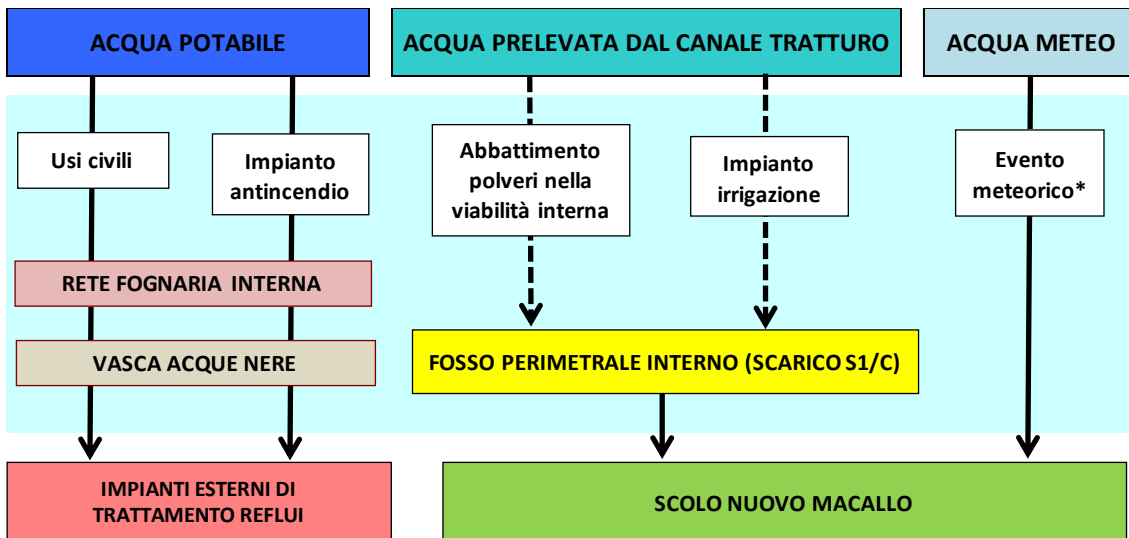
Figura 43 Ciclo idrico della discarica
