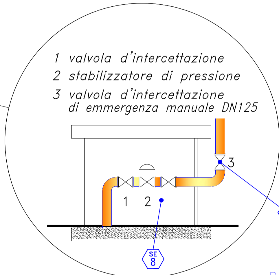
PARTICOLARE CABINA DI REGOLAZIONE DELLA PRESSIONE
