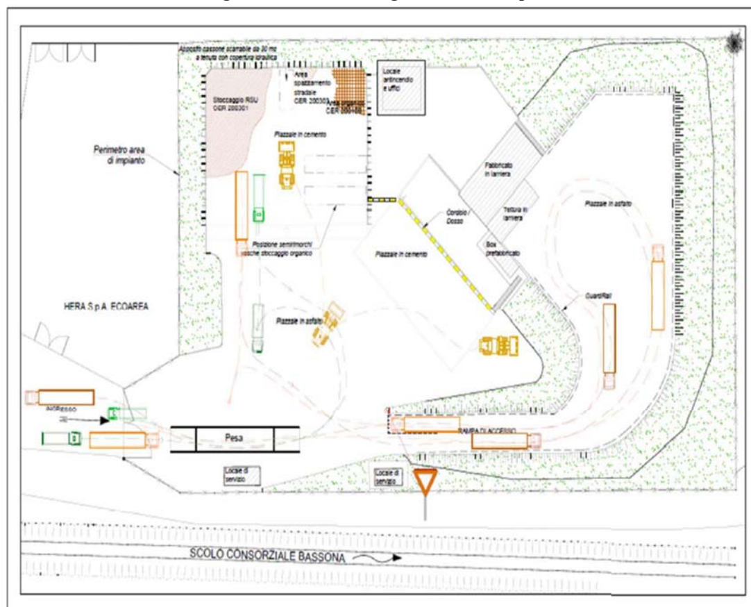
Figura 1 – Planimetria generale dell’Impianto
