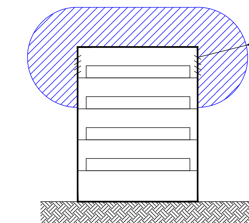
TIPICO SE 1.25 AREA CLASSIFICATA BATTERIE DA TRAZIONE
