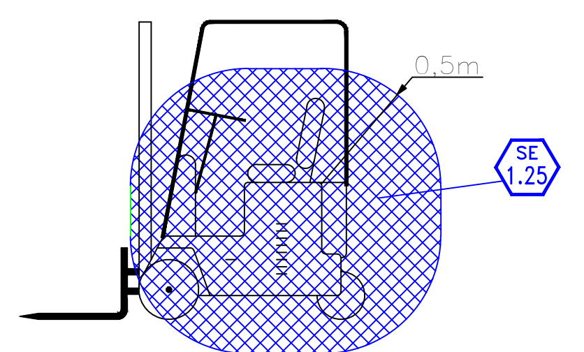
TIPICO SE 1.25 AREA CLASSIFICATA BATTERIE DA TRAZIONE
