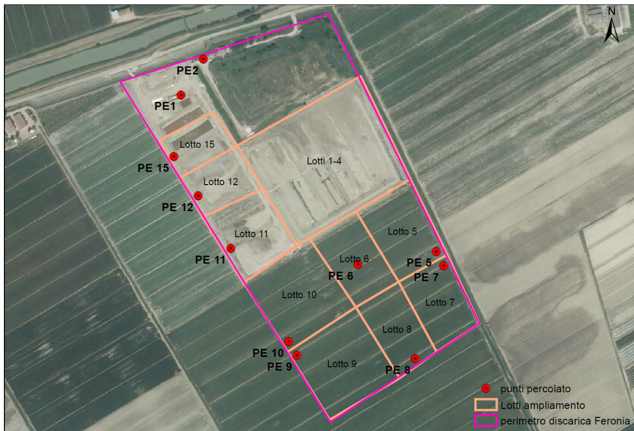
Figura 3 - Planimetria Discarica Feronia di Finale Emilia con rete di monitoraggio delle acque di percolazione.
