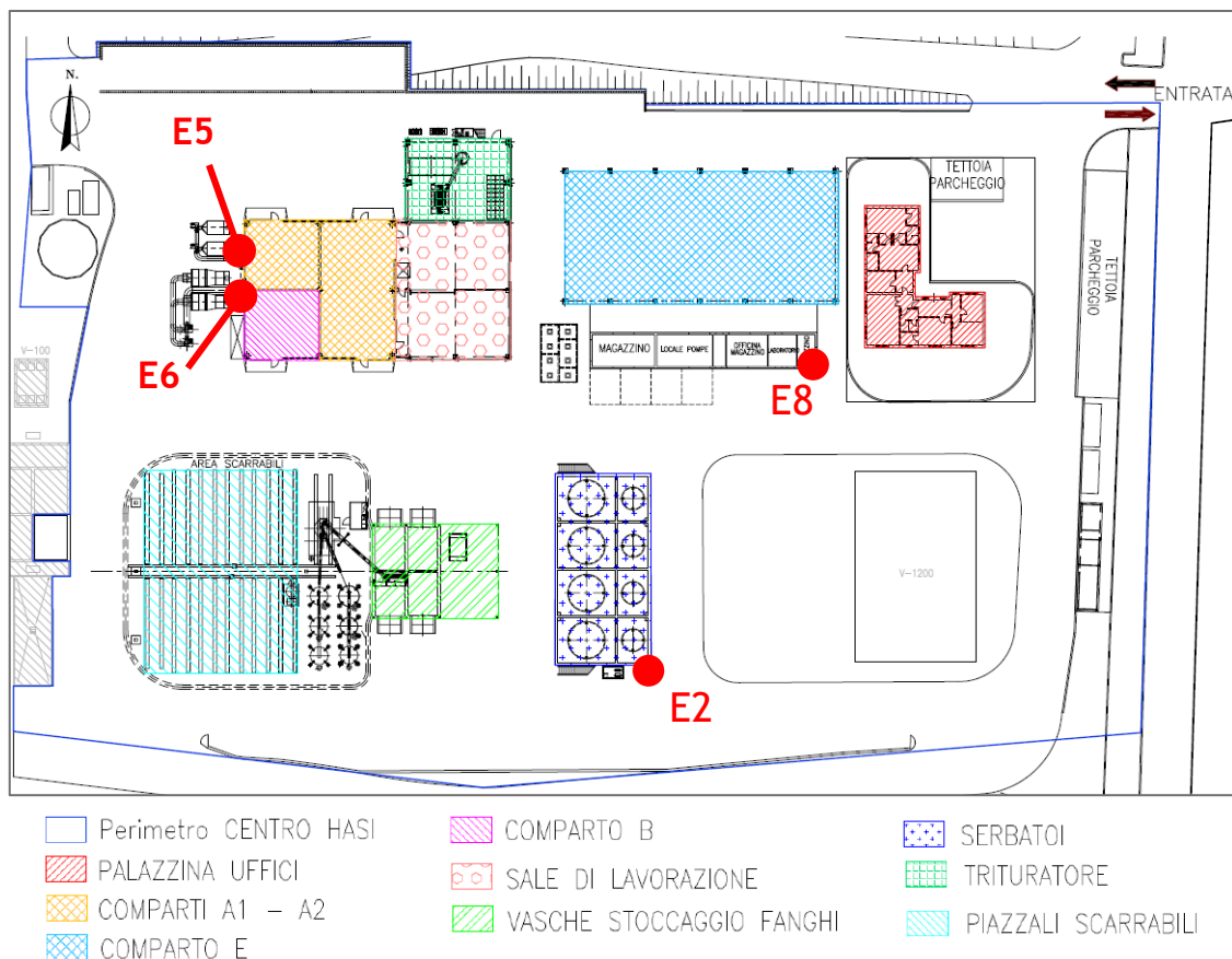
Figura 20 Localizzazione dei punti di emissione in atmosfera
