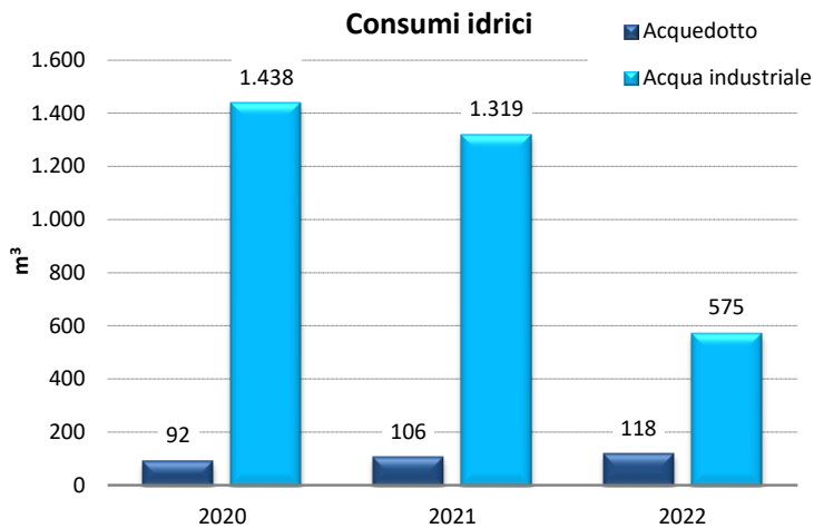
Figura 17 Andamento temporale dei consumi idrici
