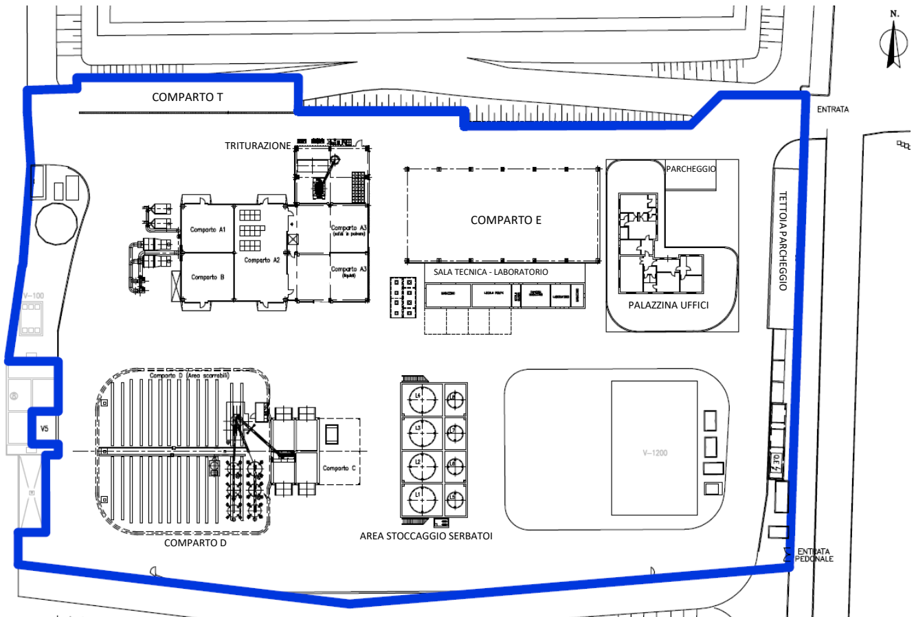
Figura 6 Planimetria del Centro di Stoccaggio e Pretrattamento rifiuti
