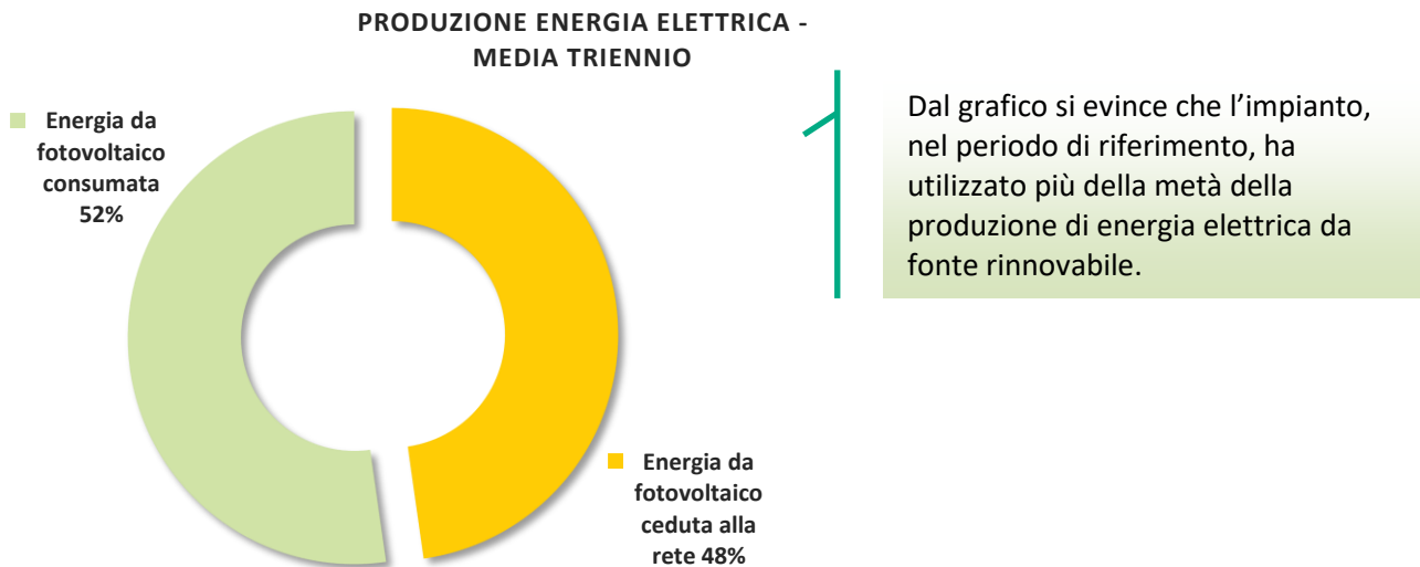
Figura 13 Ripartizione della produzione di energia da fotovoltaico (media periodo 2020-2022)
