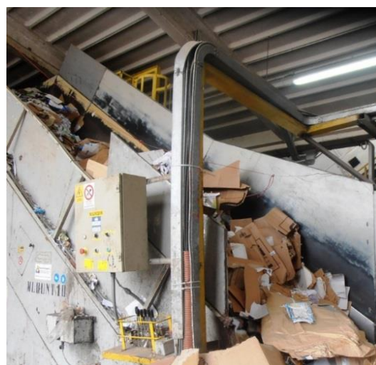
Figura 9 Particolare della pressa
