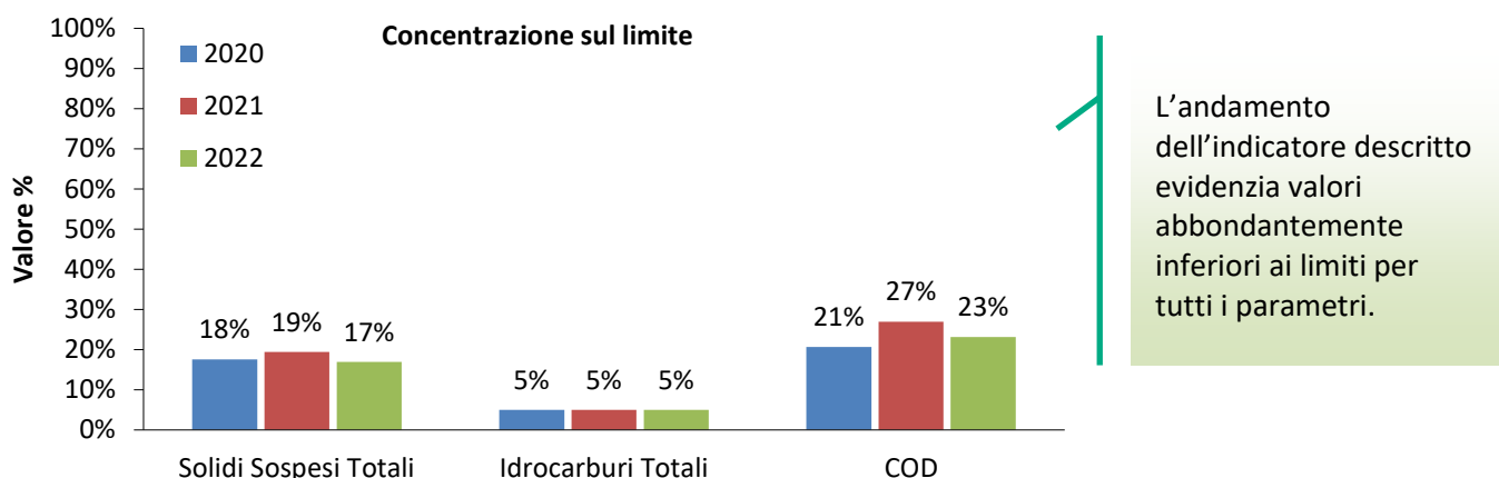
Figura 18 Andamento dell'indicatore "Posizionamento rispetto al Limite"
