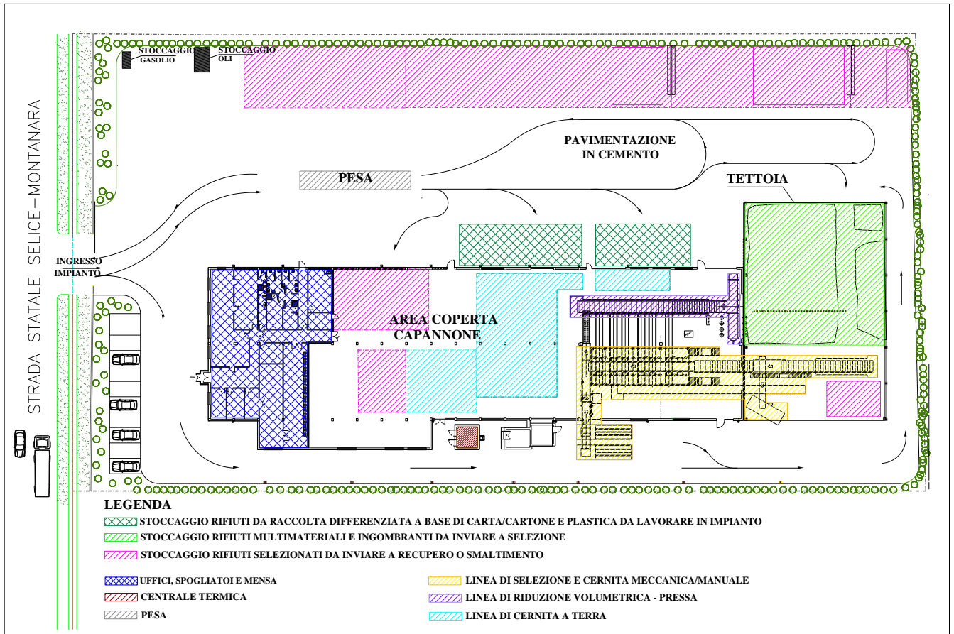
Figura 2 Planimetria del sito
