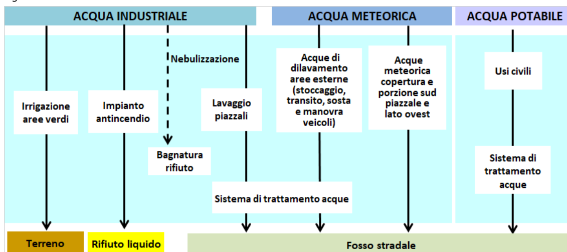
Figura 16 Ciclo idrico
