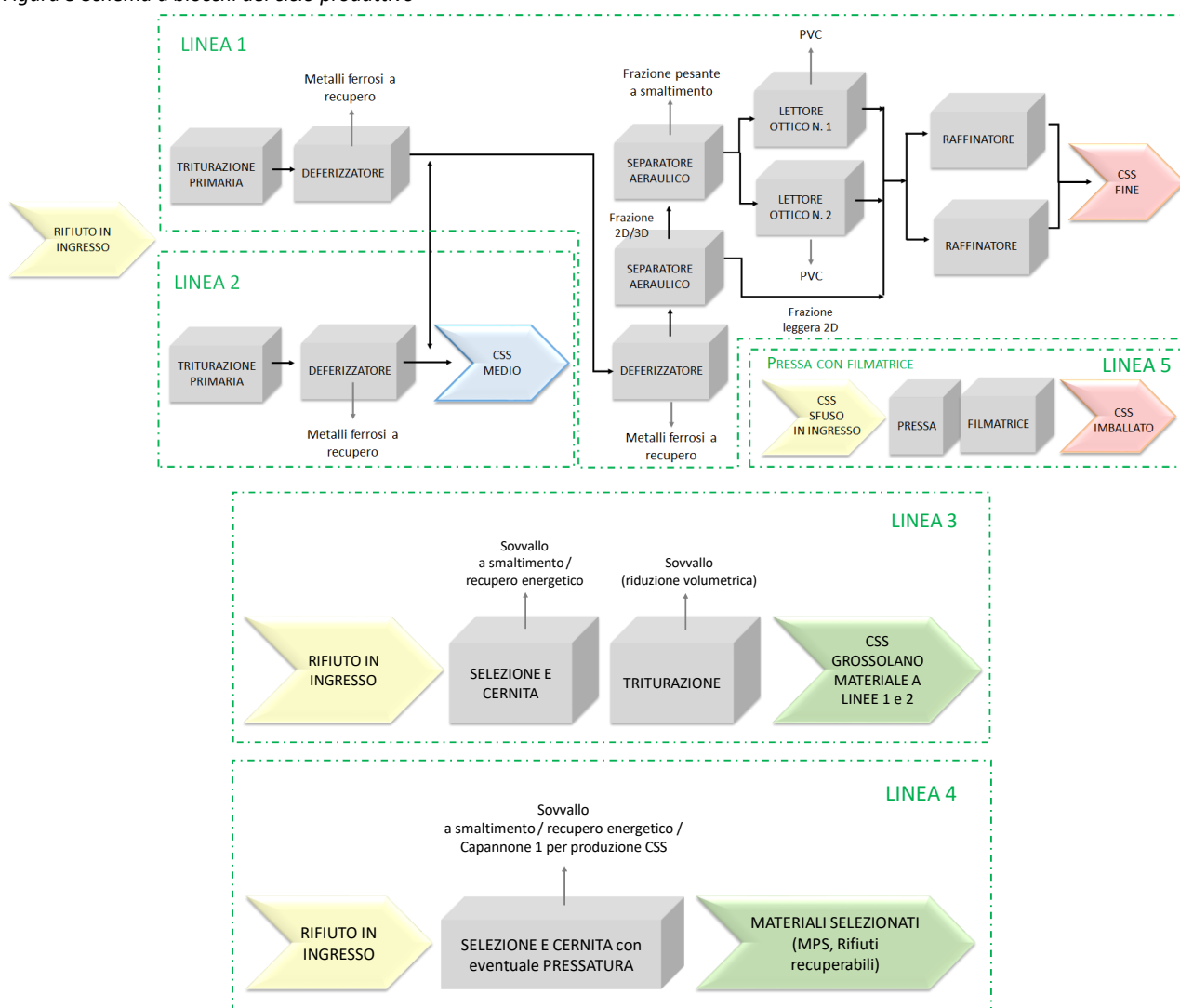
Figura 5 Schema a blocchi del ciclo produttivo
