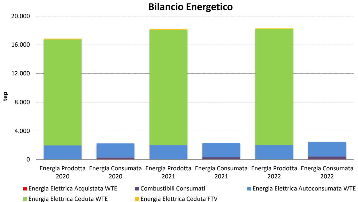
Figura 9 Bilancio energetico del complesso impiantistico in tep (Energia prodotta / consumata)
