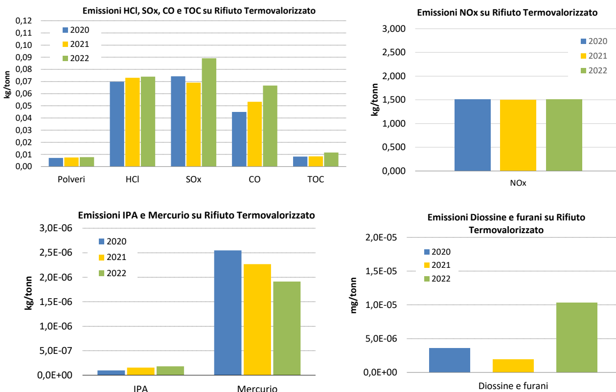
Figura 17 Andamento dell'indicatore "Fattori di Emissione Specifici"
