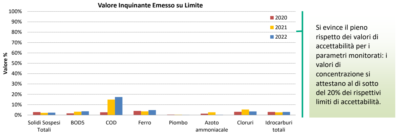
Figura 15 Andamento dell'indicatore "Posizionamento Rispetto al Limite"
