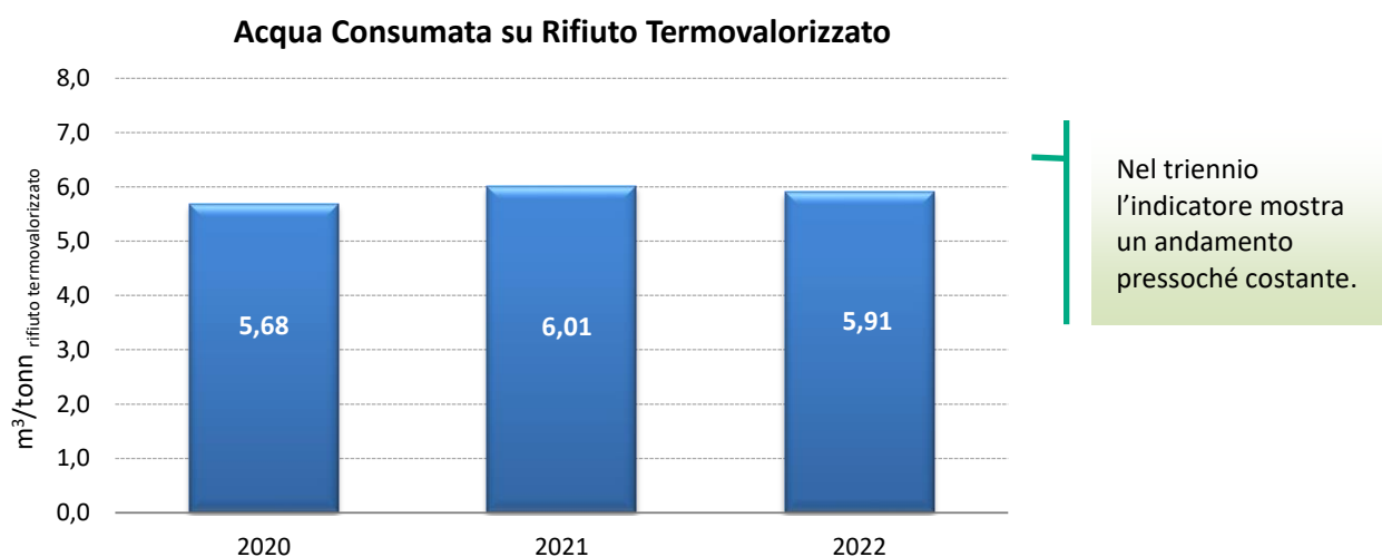
Figura 13 Indicatore "Efficienza di Utilizzo della Risorsa Idrica"
