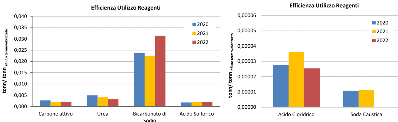
Figura 19 Andamento dell'indicatore "Fattore di utilizzo reagenti"
