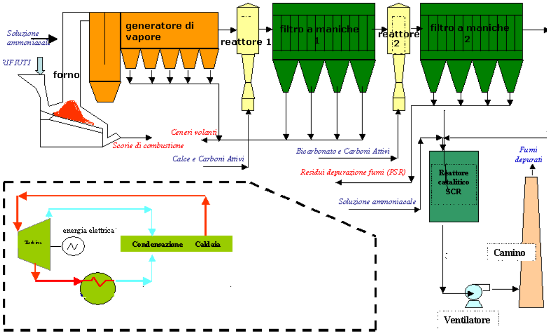
Figura 6 Ciclo produttivo del termovalorizzatore
