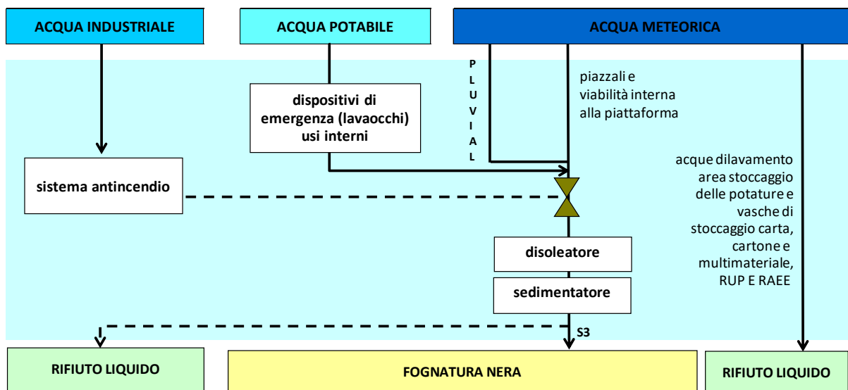
Figura 30 Ciclo idrico della piattaforma ecologica
