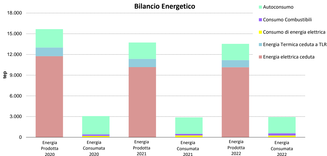
Figura 24 Bilancio energetico del termovalorizzatore
