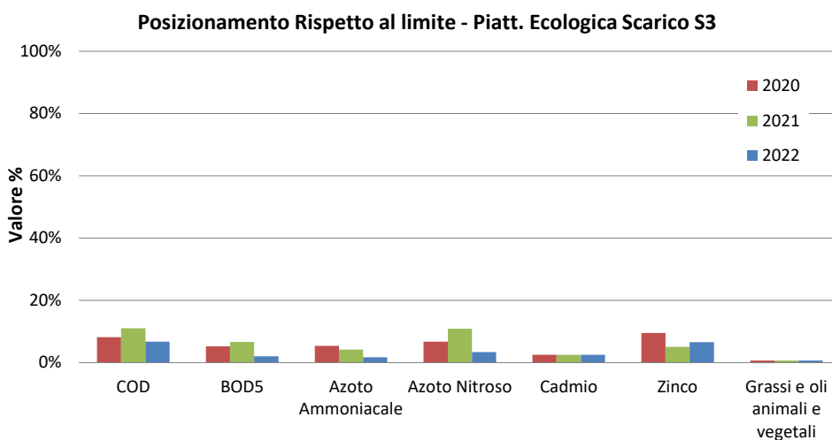
Figura 33 Andamento dell'indicatore "Posizionamento Rispetto al Limite" (S3)
