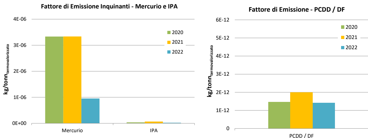
Figura 39 Andamento dell'indicatore "Fattori di Emissione Microinquinanti"
