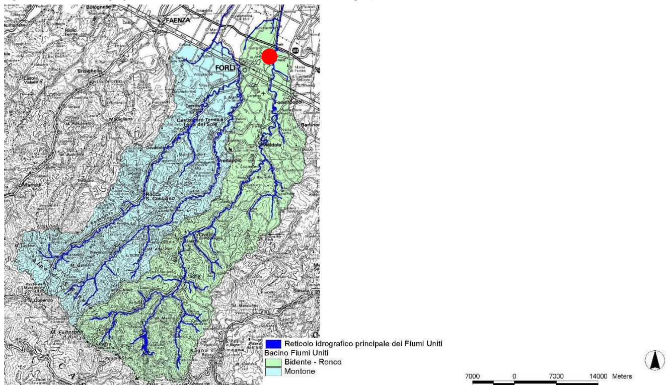
Figura 2 Reticolo idrografico dei Fiumi Uniti (Fonte: ARPAE Emilia-Romagna)
