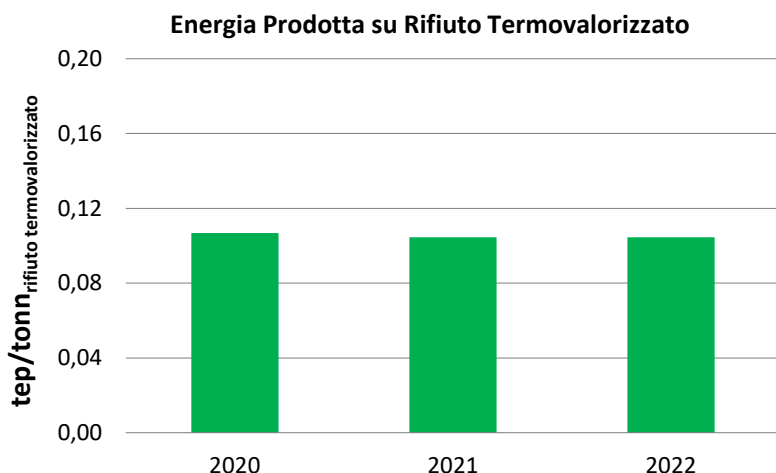
Figura 27 Andamento dell'indicatore "Energia Recuperata dal Rifiuto"
