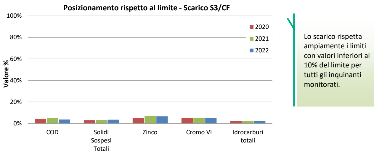
Figura 34 Andamento dell'indicatore "Posizionamento Rispetto al Limite" (S3/CF)
