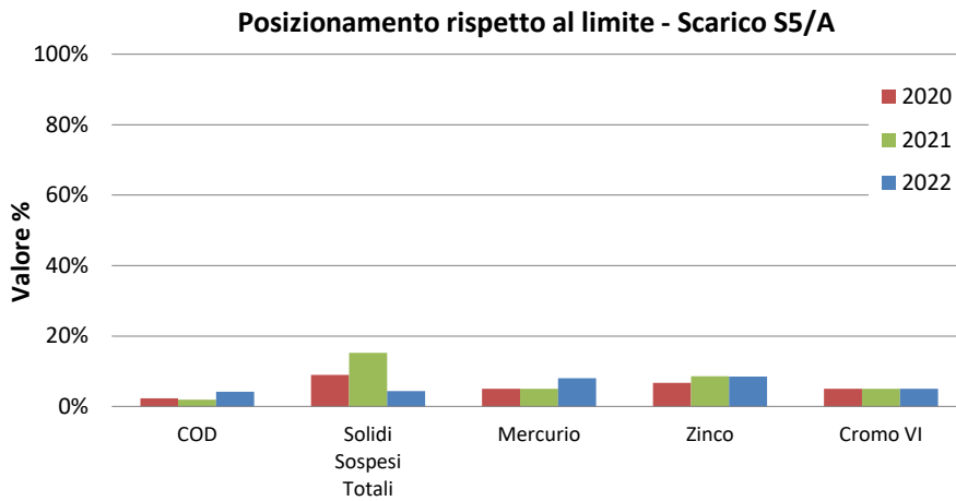
Figura 32 Andamento dell'indicatore "Posizionamento Rispetto al Limite" (S5/A)
