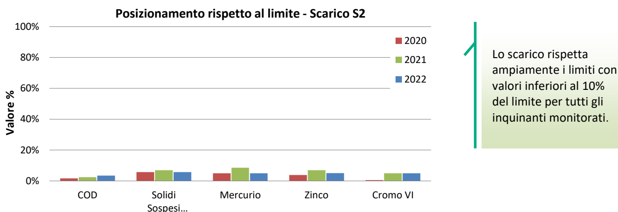
Figura 31 Andamento dell'indicatore "Posizionamento Rispetto al Limite" (S2)
