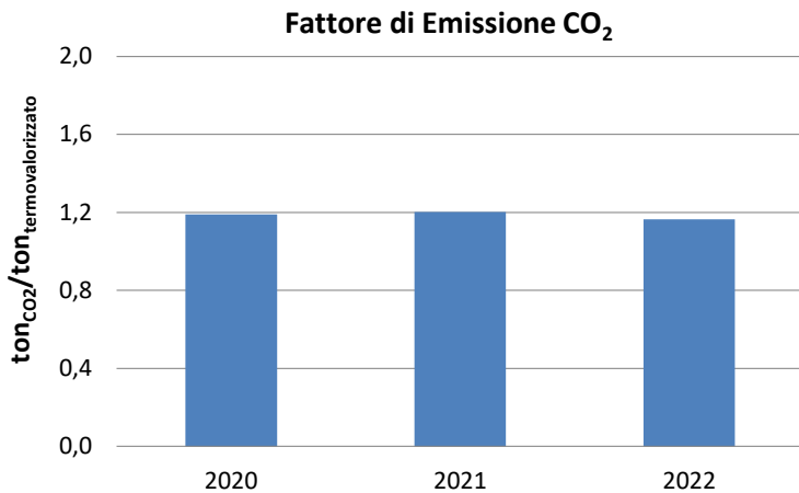
Figura 42 Andamento dell'indicatore "Fattori di emissione dei gas serra"
