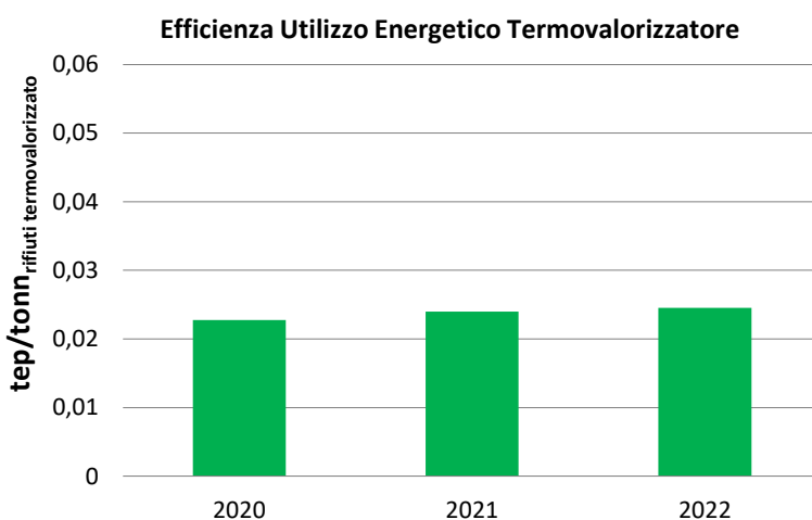
Figura 26 Andamento dell'indicatore "Efficienza di Utilizzo Energetico"
