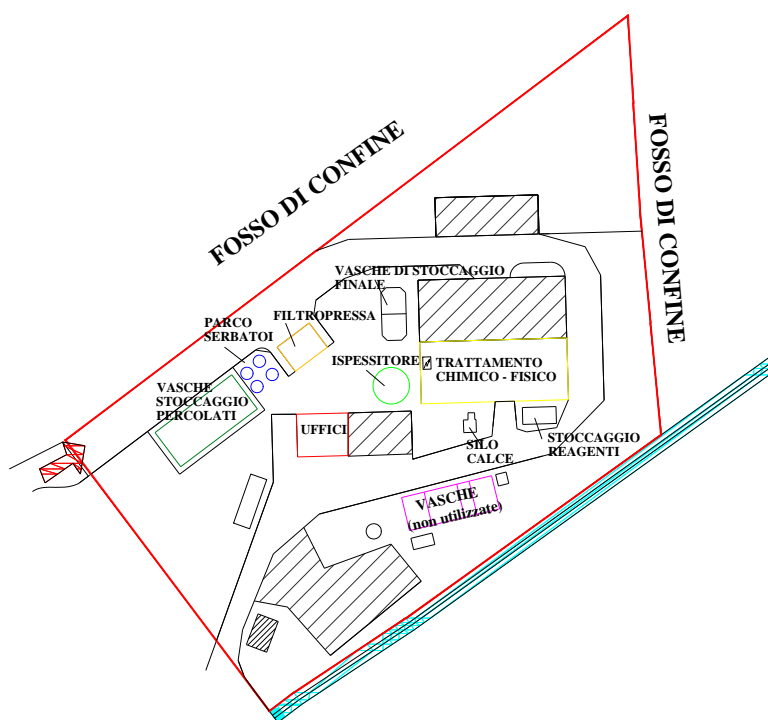
Figura 4 Particolare dell'impianto chimico-fisico
