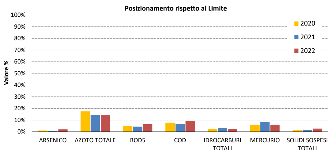
Figura 17 Andamento dell'indicatore "Posizionamento rispetto al Limite" - Scarico S1
