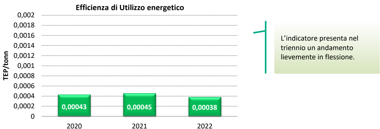
Figura 13 Andamento dell’indicatore “Efficienza di utilizzo energetico”
