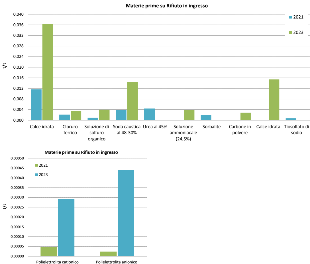
Figura 44 Andamento dell'indicatore "Fattore di utilizzo reagenti" (F3)
