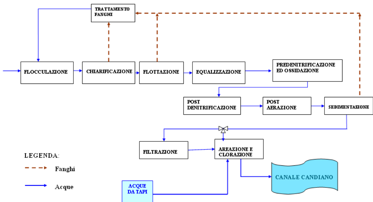
Figura 13 Ciclo produttivo (TAPO)
