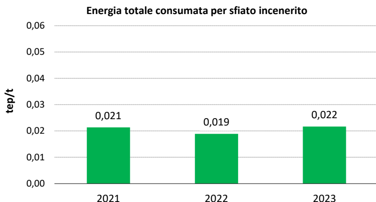
Figura 25 Andamento dell'indicatore "Efficienza di utilizzo energetico" (FIS)
