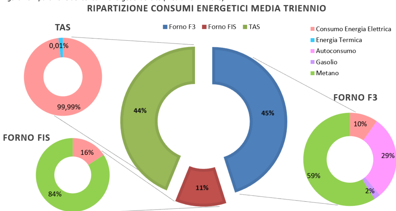
Figura 20 Ripartizione dei consumi energetici del sito (media 2021 - 2023)
