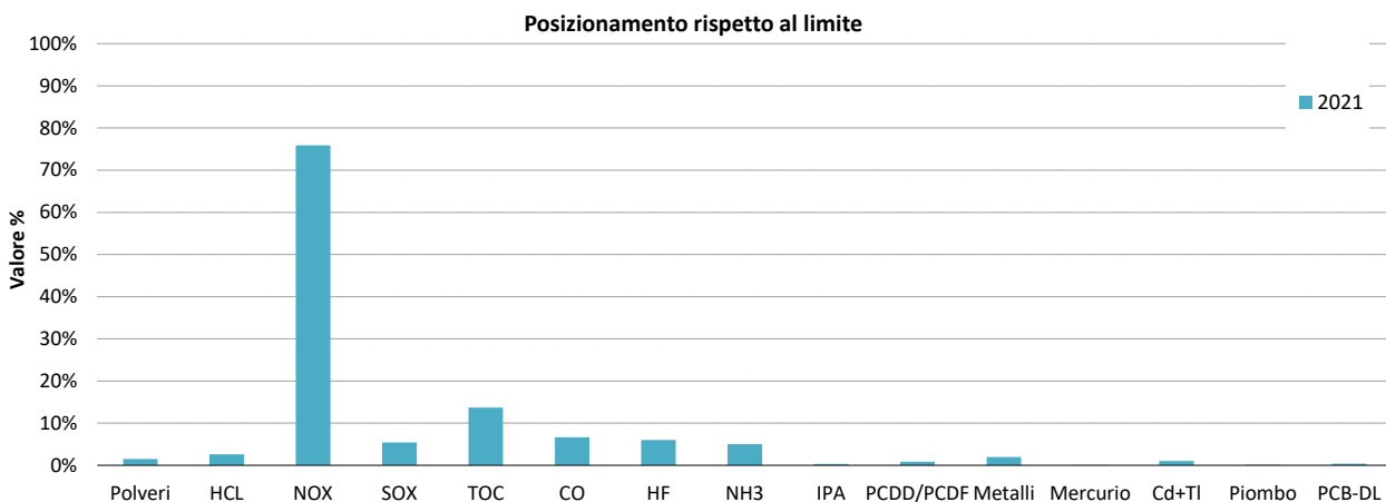
Figura 38 Andamento dell'indicatore "Posizionamento rispetto al limite" (E3)
