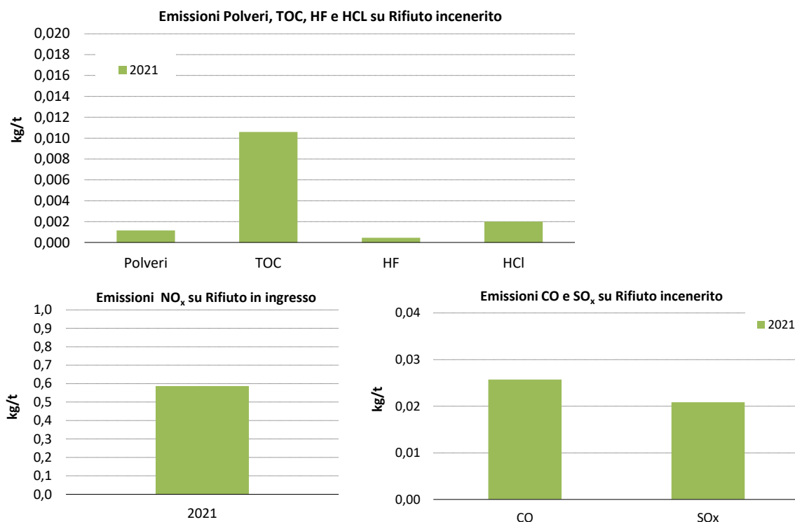
Figura 39 Andamento dell'indicatore "Fattori di emissione specifici" (E3)
