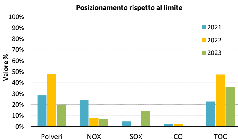
Figura 42 Andamento dell'indicatore "Posizionamento rispetto al Limite" (E4)
