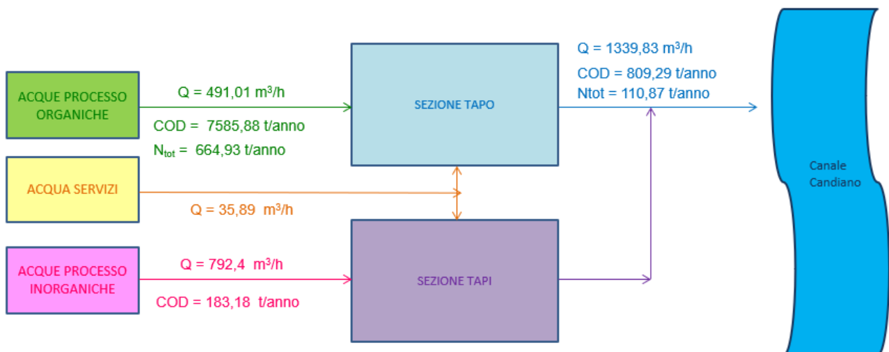
Figura 36 Bilancio impianto TAS (2023)
