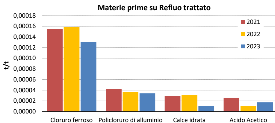
Figura 45 Andamento dell'indicatore "Fattore di utilizzo reagenti" (TAS)
