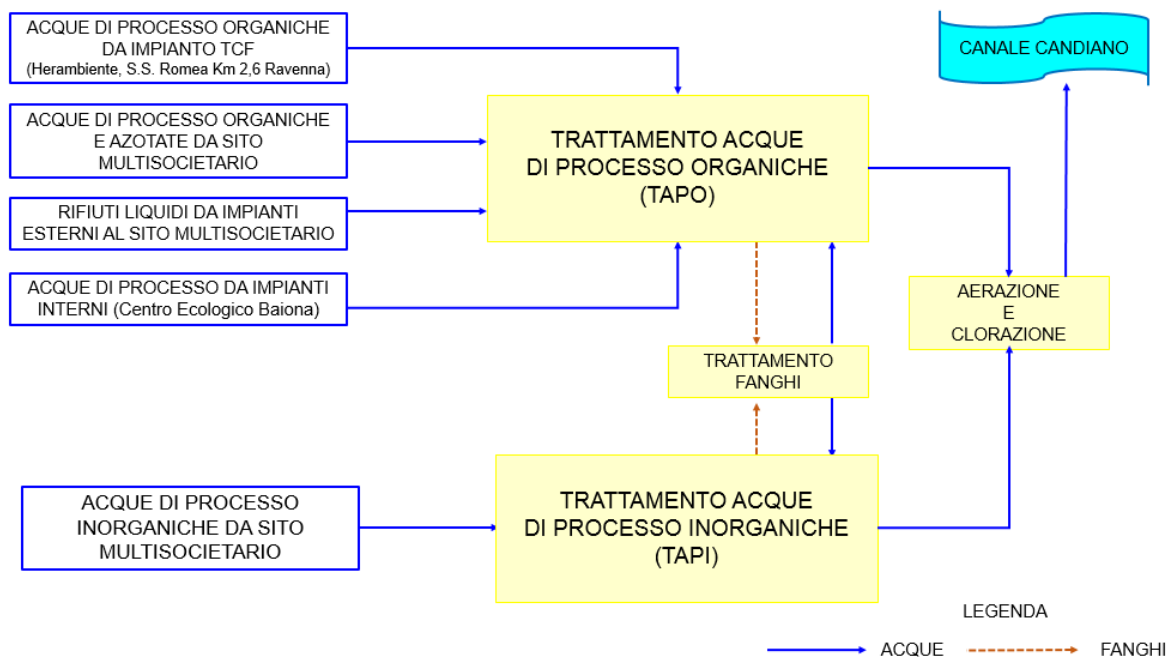
Figura 12 Ciclo produttivo (TAS)
