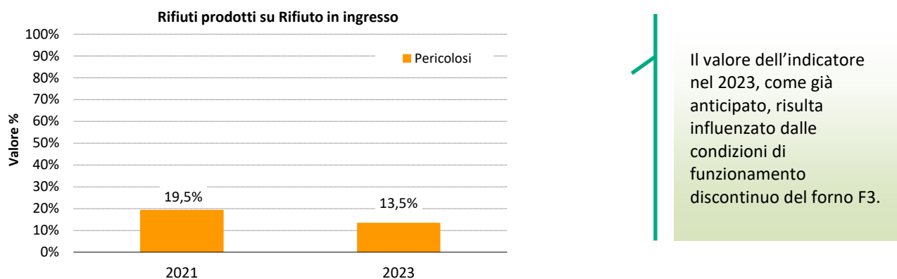
Figura 47 Andamento dell'indicatore "Rifiuto autoprodotta su Rifiuto in ingresso" (F3)
