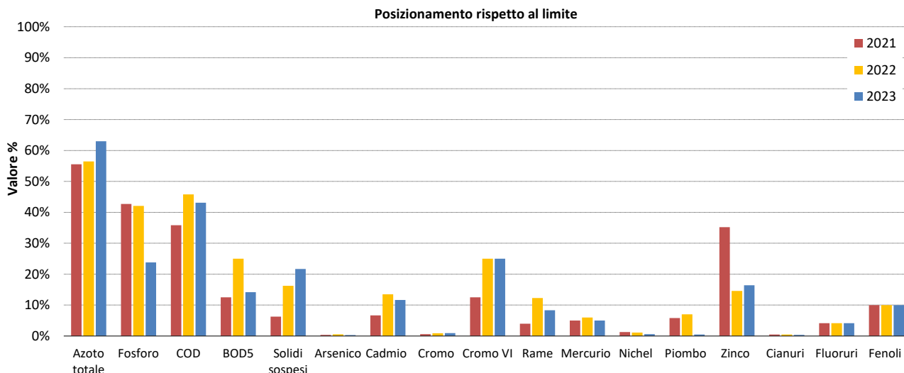
Figura 34 Andamento dell'indicatore "Posizionamento rispetto al limite"
