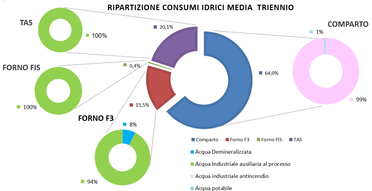
Figura 27 Ripartizione dei consumi idrici di comparto (media 2021 - 2023)
