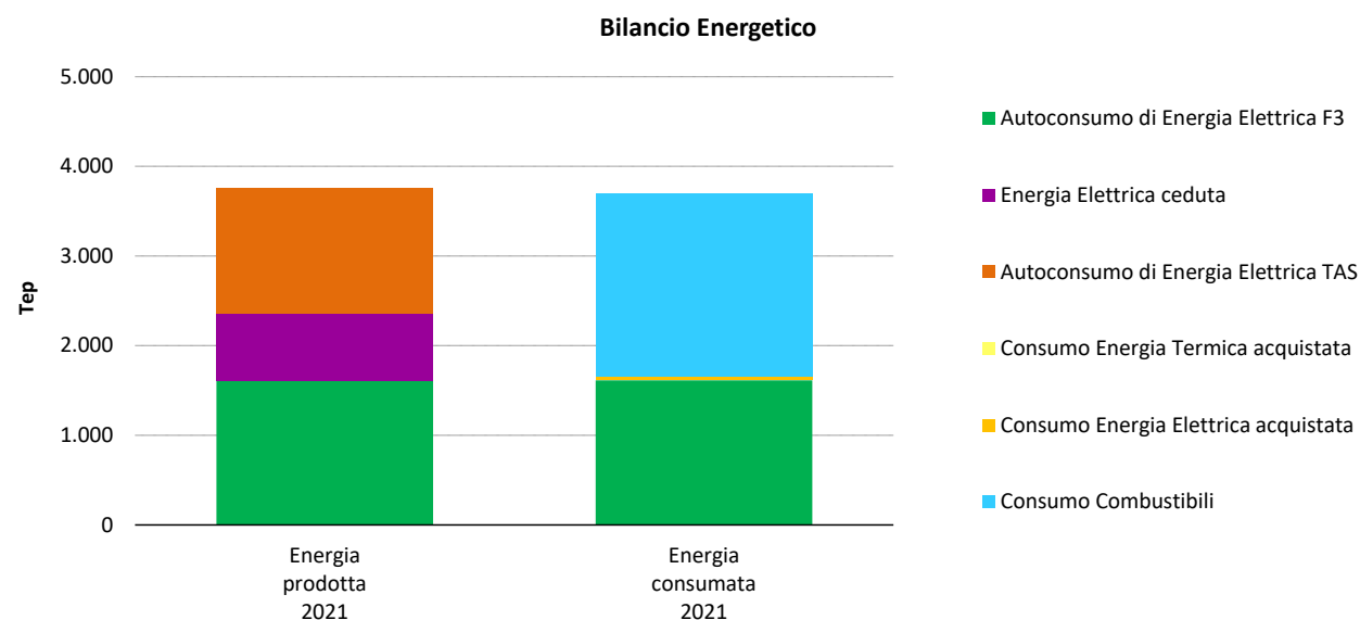
Figura 22 Bilancio energetico del termovalorizzatore (F3)
