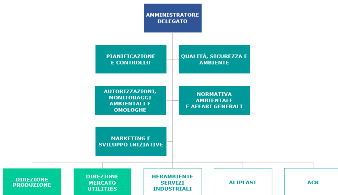
Organigramma aziendale
