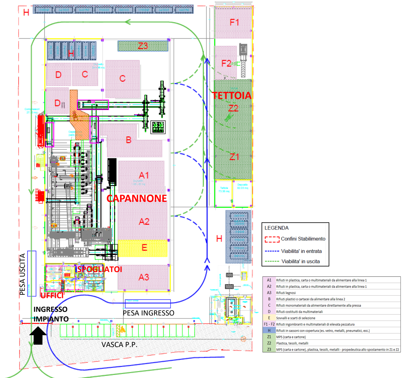
Figura 3 Planimetria del sito
