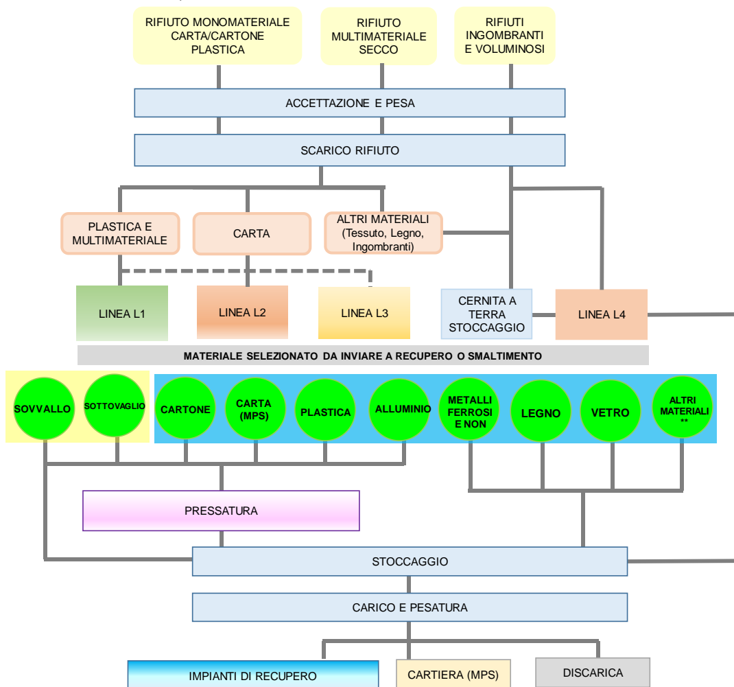
Figura 7 Schema a blocchi del ciclo produttivo
