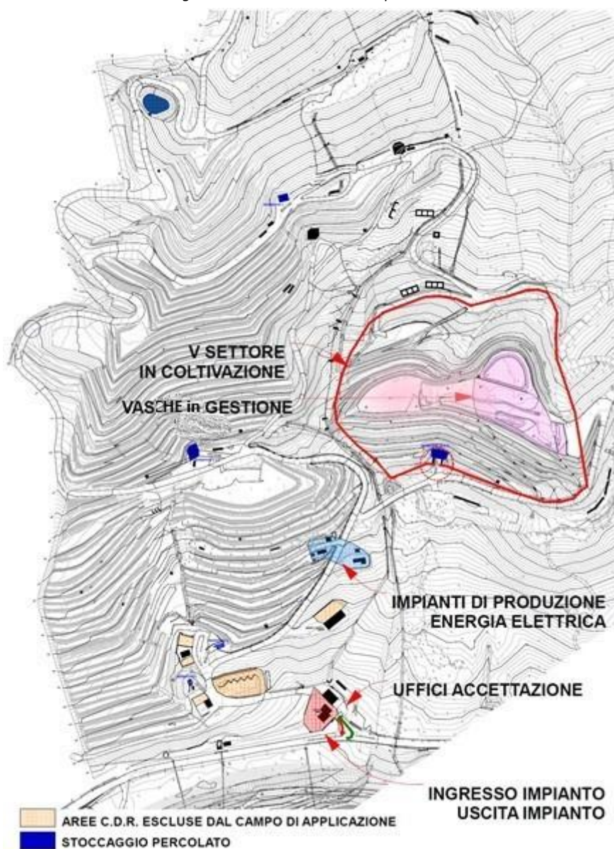
Figura 1 Planimetria del sito impiantistico
