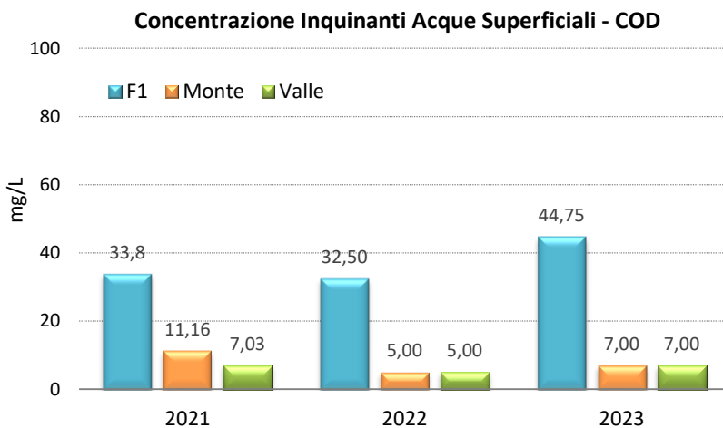
Figura 15 Andamento concentrazione COD triennio 2021-2023
