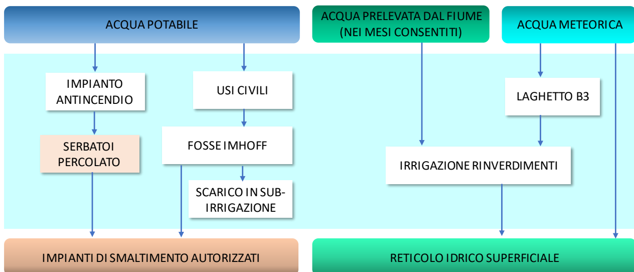
Figura 12 Ciclo idrico
