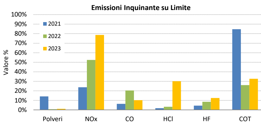
Figura 17 Indicatore "Posizionamento rispetto al Limite" – E1
