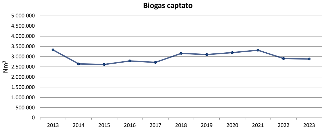
Figura 8 Andamento temporale del quantitativo di biogas estratto dal corpo discarica
