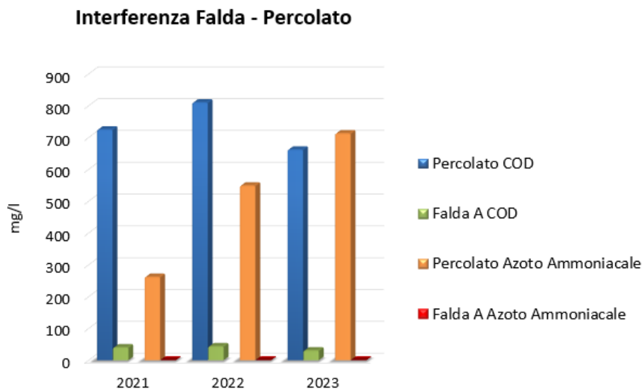
Figura 23 Confronto tra gli andamenti dei markers nel percolato e nella falda A di primo livello
