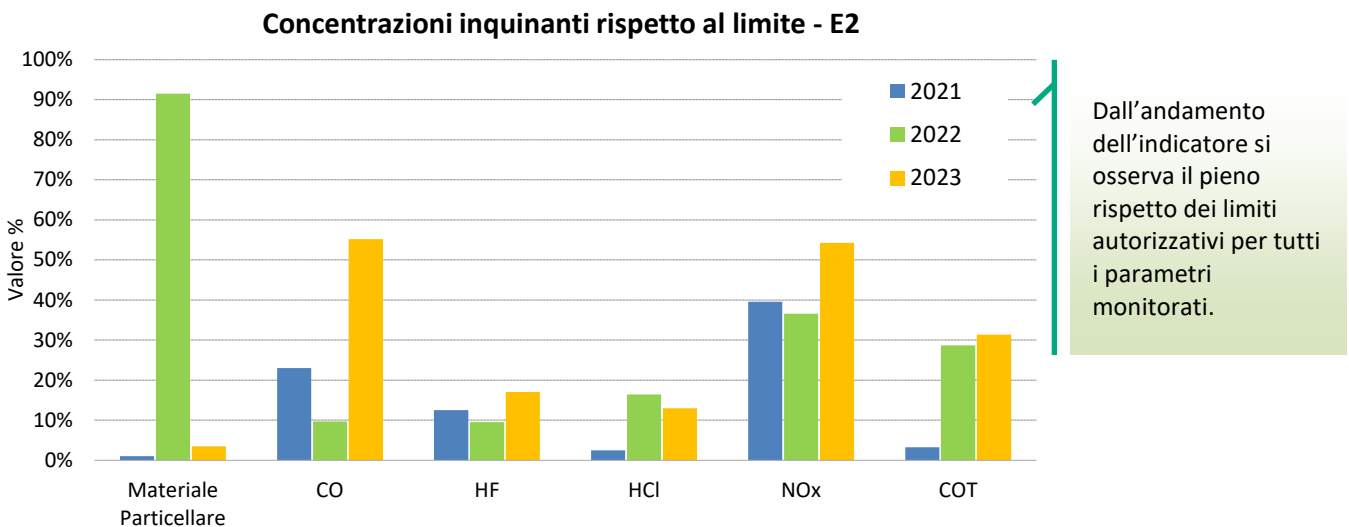
Figura 25 Andamento dell'indicatore "Posizionamento rispetto al limite" (E2)
