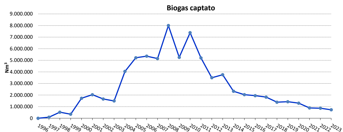
Figura 12 Quantitativi di biogas estratto durante il ciclo di vita della discarica
