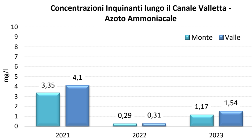
Figura 18 Confronto Azoto ammoniacale a monte e a valle del sito
