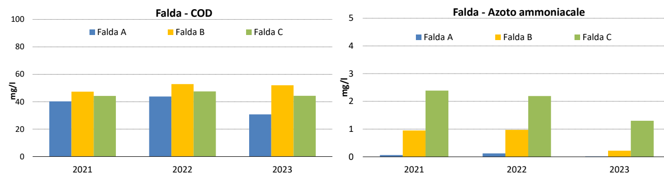
Figura 22 Andamento del COD e dei markers per le acque di falda
