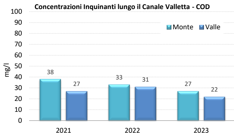
Figura 19 Confronto COD a monte e a valle del sito verificare grafico
