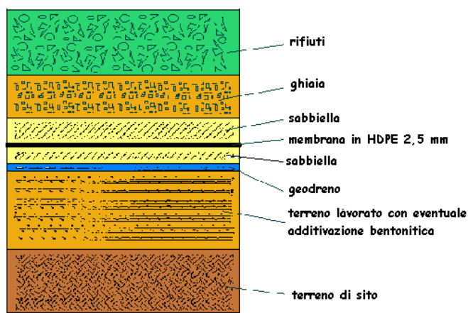
Figura 20 Struttura del fondo della discarica
