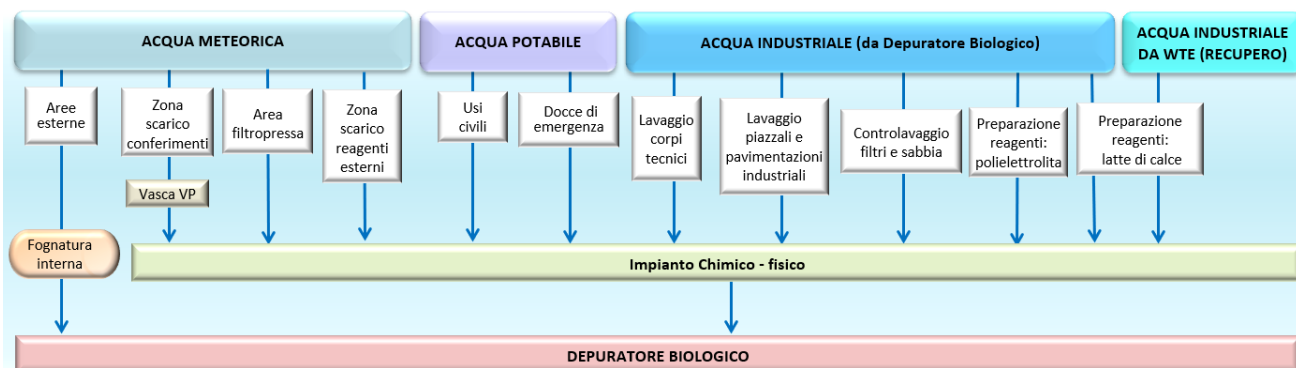
Figura 24 Ciclo idrico dell’impianto chimico-fisico
