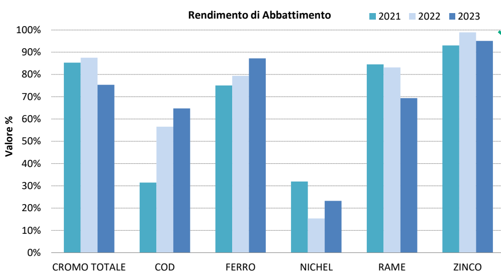
Figura 28 Rendimenti di abbattimento
