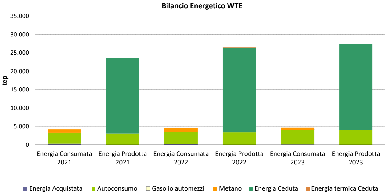
Figura 17 Bilancio energetico del termovalorizzatore
