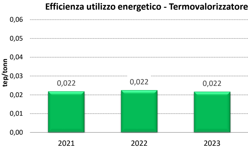
Figura 19 Andamento dell'indicatore "Efficienza di utilizzo energetico"
