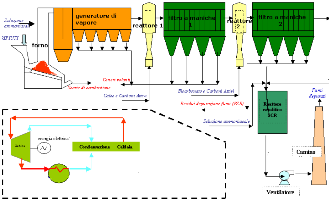
Figura 6 Ciclo produttivo del termovalorizzatore
