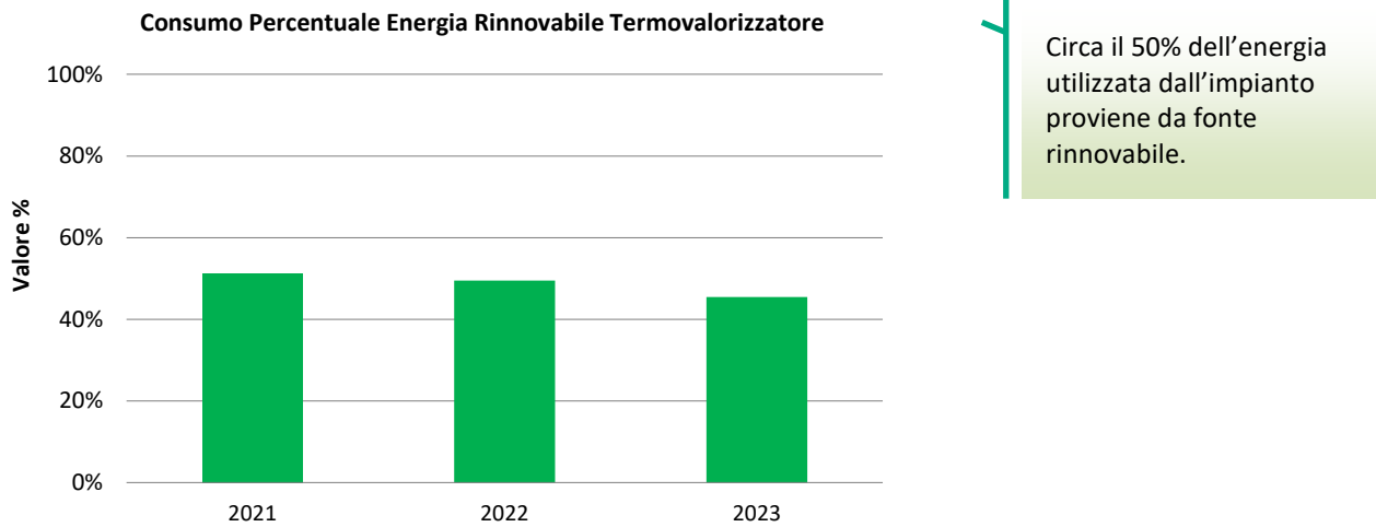
Figura 25 Andamento dell'indicatore "Utilizzo di Energia da Fonte Rinnovabile"
