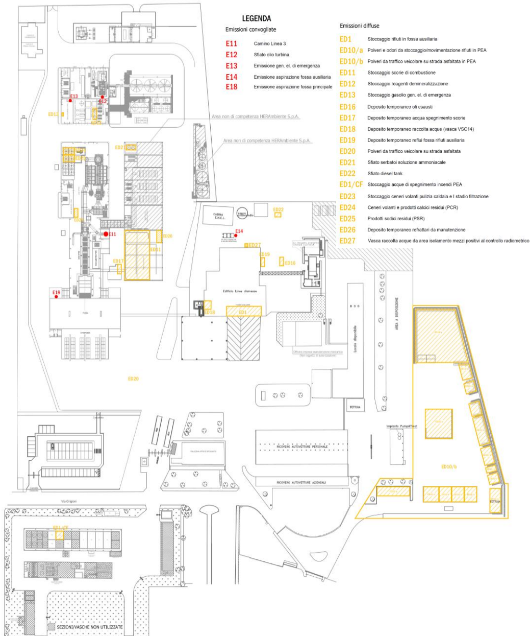
Figura 35 Planimetria delle emissioni del sito
