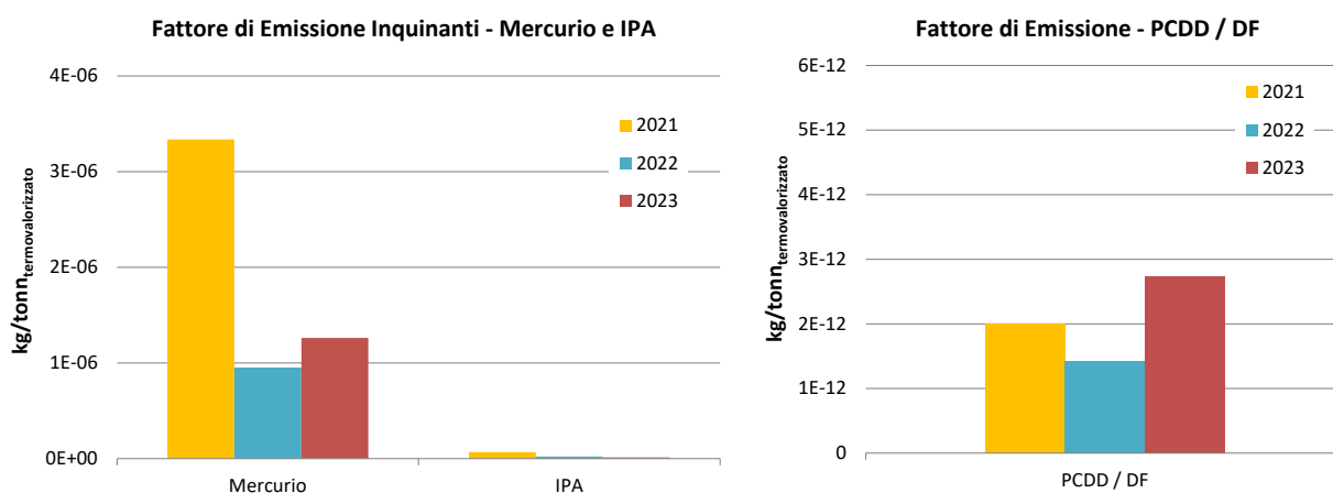
Figura 39 Andamento dell'indicatore "Fattori di Emissione Microinquinanti"
