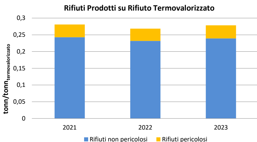
Figura 46 Andamento dell'indicatore "Rifiuto autoprodotta su rifiuto termovalorizzato"
