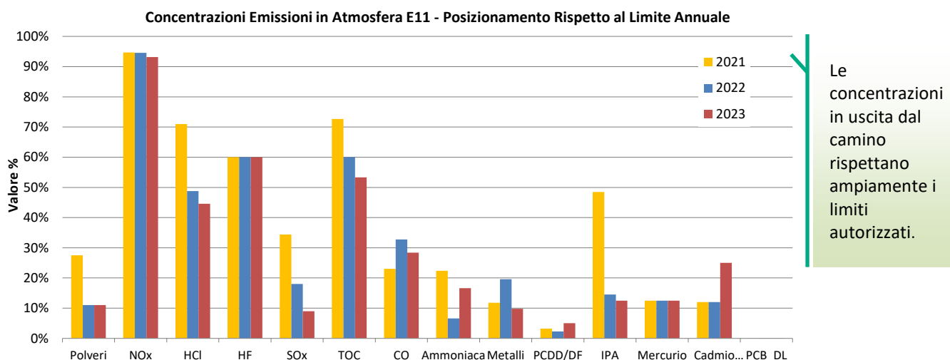
Figura 37 Andamento dell'indicatore "Posizionamento Rispetto al Limite"
