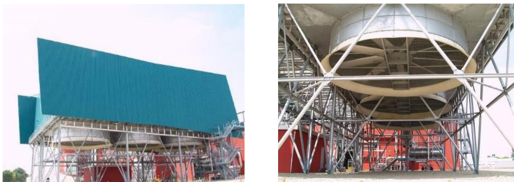
Figura 12 Particolari del condensatore
