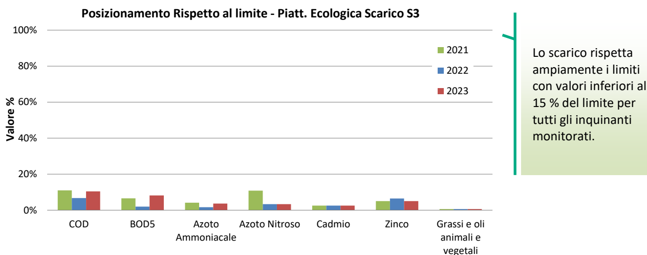
Figura 33 Andamento dell'indicatore "Posizionamento Rispetto al Limite" (S3)
