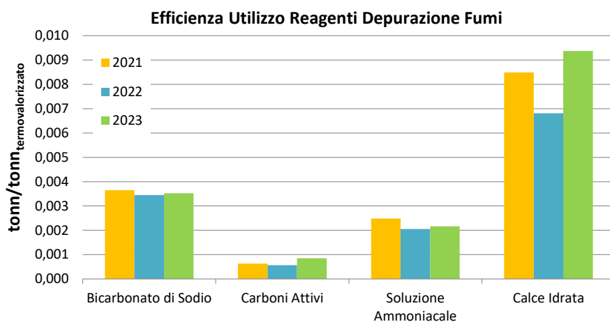
Figura 43 Andamento dell'indicatore "Fattore di utilizzo reagenti"
