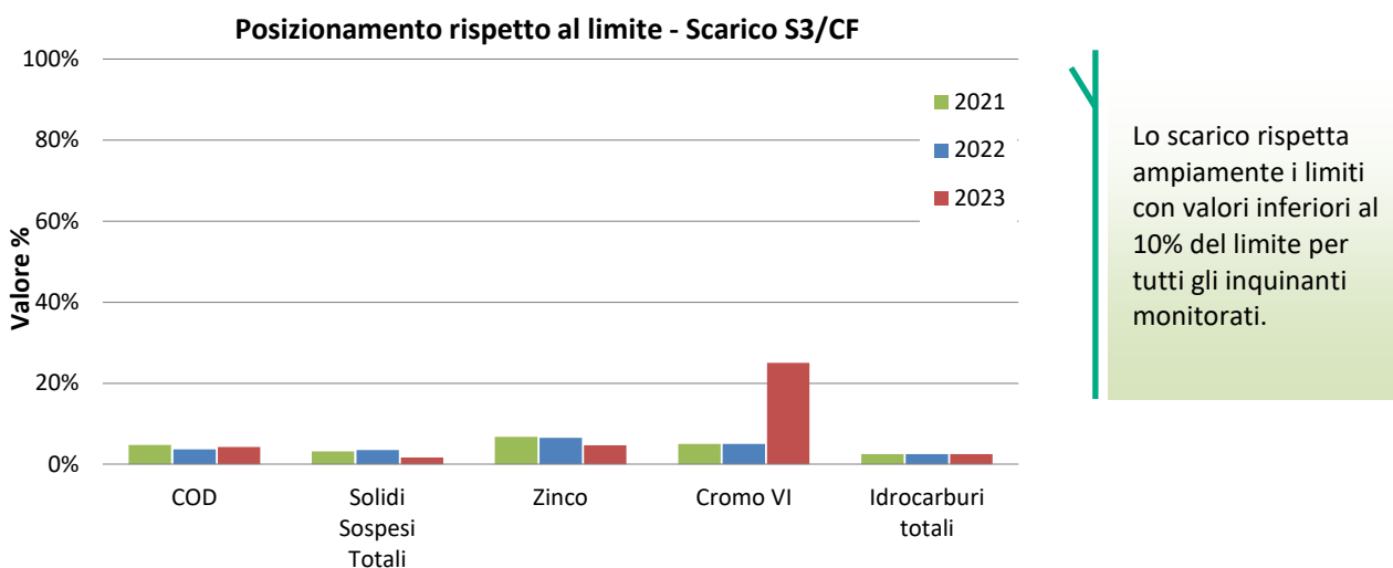
Figura 34 Andamento dell'indicatore "Posizionamento Rispetto al Limite" (S3/CF)
