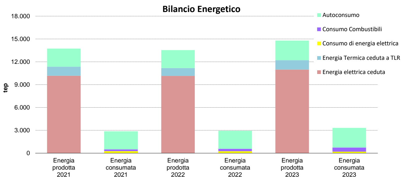
Figura 24 Bilancio energetico del termovalorizzatore
