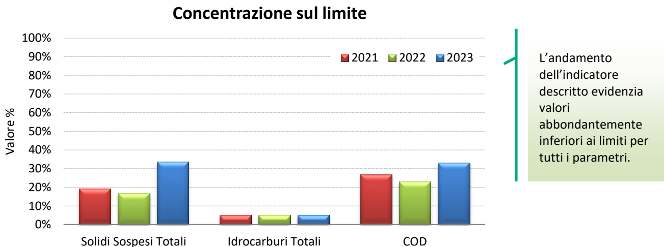
Figura 18 Andamento dell'indicatore "Posizionamento Rispetto al Limite"
