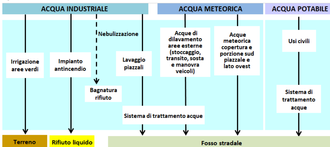
Figura 16 Ciclo idrico
