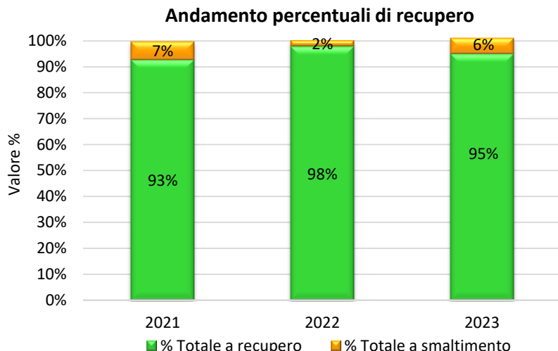
Figura 20 Andamento percentuali di recupero e smaltimento rispetto ai rifiuti in ingresso all'impianto di selezione
