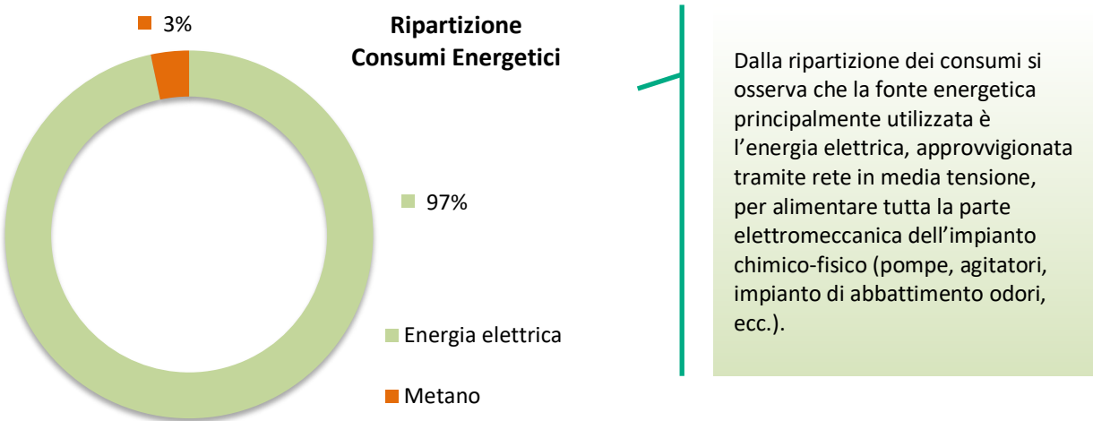
Figura 12 Composizione media dei consumi energetici (media triennio 2022 - 2024)
