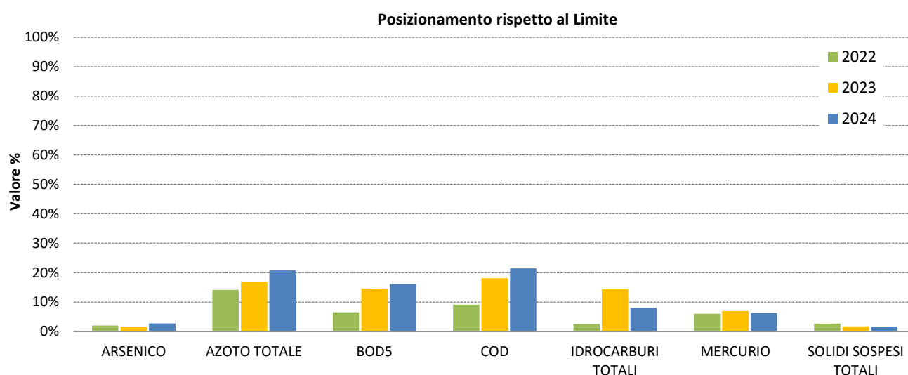
Figura 17 Andamento dell'indicatore "Posizionamento rispetto al Limite" - Scarico S1
