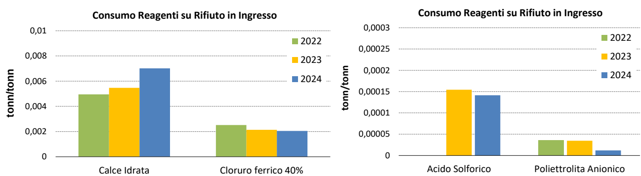
Figura 20 Andamento dell’indicatore “Fattore di utilizzo reagenti”
