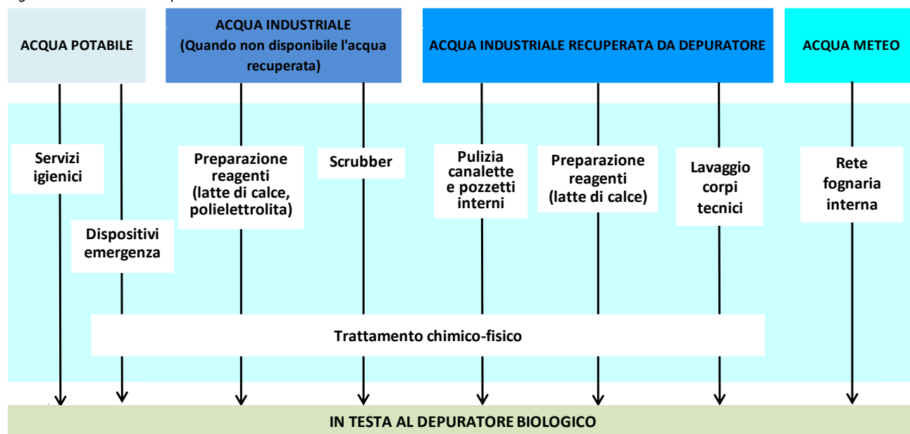
Figura 14 Ciclo idrico Impianto
