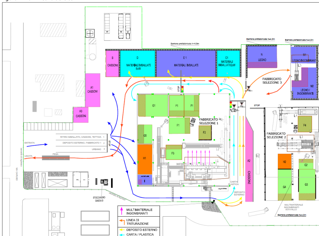
Figura 4 Planimetria del sito
