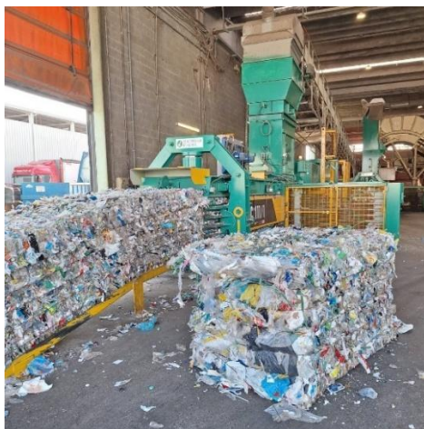
Figura 11 Pressa linea L2
