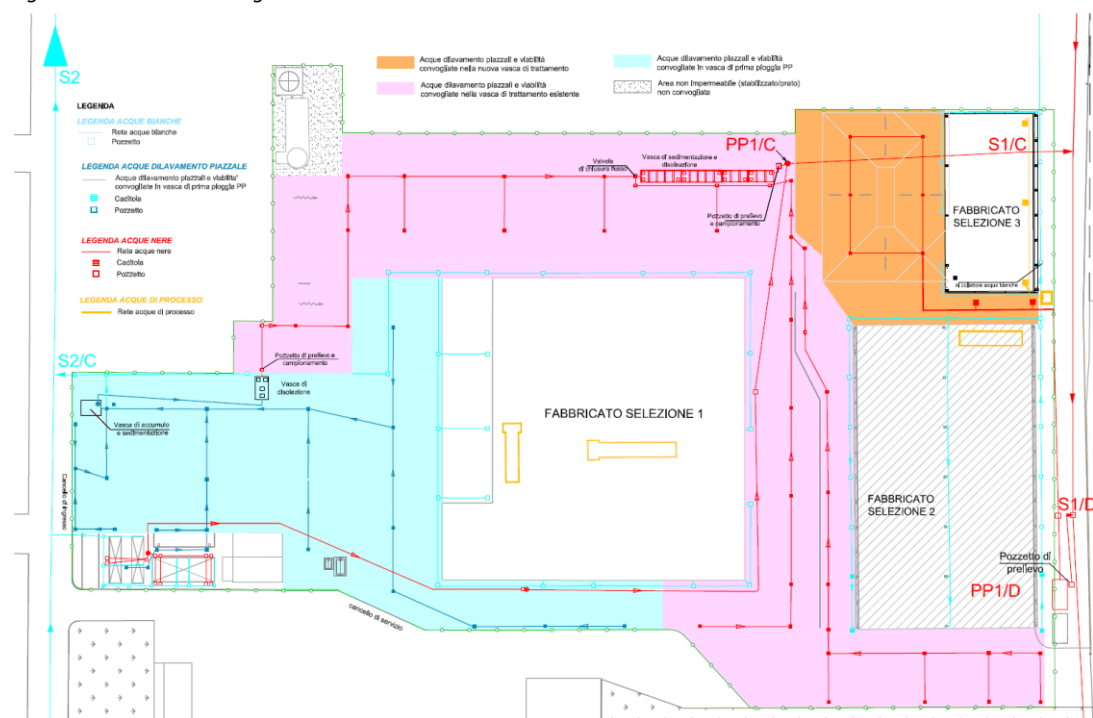
Figura 21 Planimetria degli scarichi idrici
