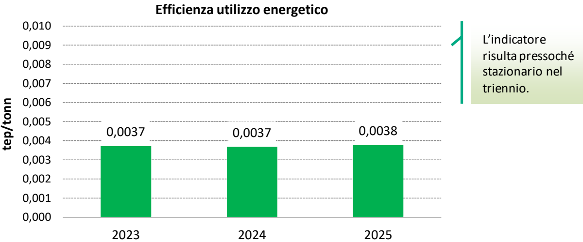
Figura 18 Andamento dell'indicatore "Efficienza di utilizzo energetico"
