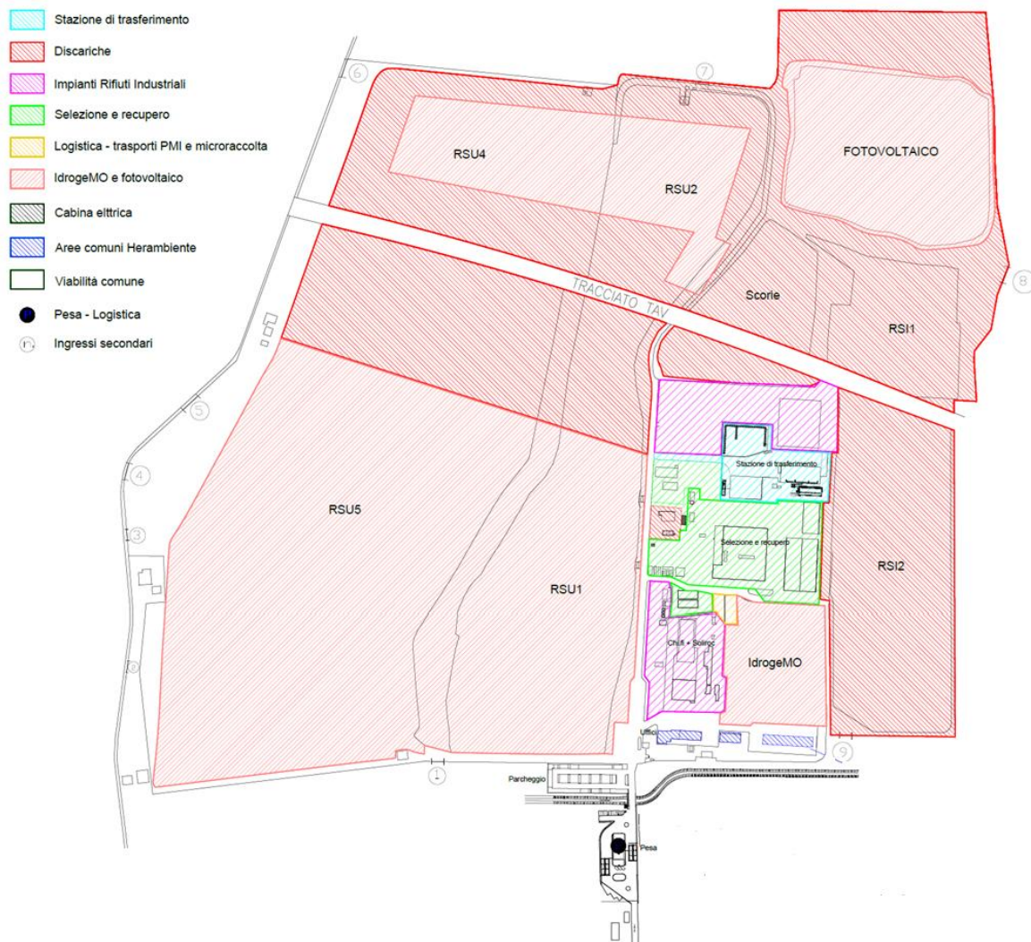
Figura 1 Planimetria del complesso impiantistico di Modena denominato "AREA 3" con le aree di competenza
