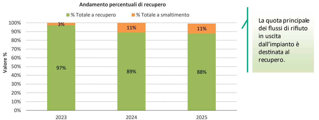
Figura 27 Andamento percentuali di recupero e smaltimento rispetto ai rifiuti in ingresso all’impianto di selezione
