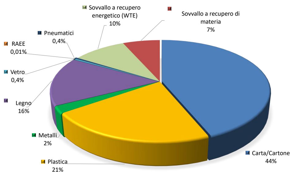
TIPOLOGIE FLUSSI IN USCITA A RECUPERO
